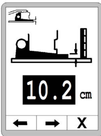
Aktuell gemessene Schichtdicke.
