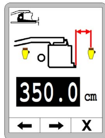
Abstand von der Mitte des ersten Sensors bis zur Mitte des zweiten Sensors.
