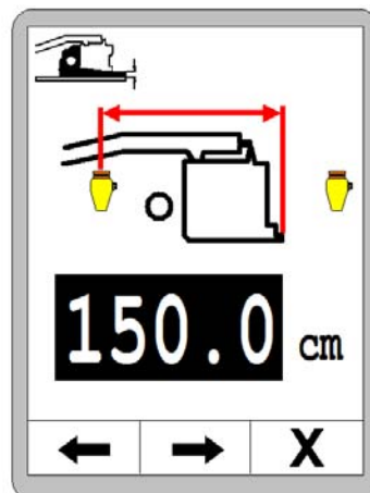
Abstand von der Bohlenhinterkante bis zur Mitte des ersten Sensors.
