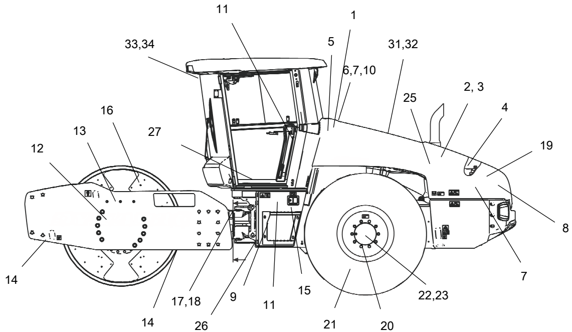
图：保养和维护部位
