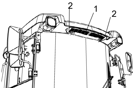
图：驾驶室 1. 新鲜空气过滤器 (x 2) 2. 螺丝 (x 3)
