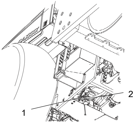
图：机器的右下方 1. 排放塞 2. 排放阀
