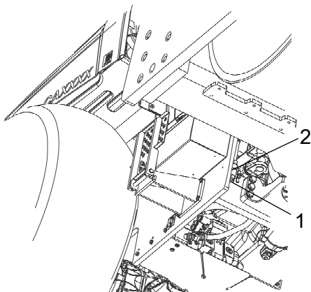
Fig. Dessous droit du rouleau
