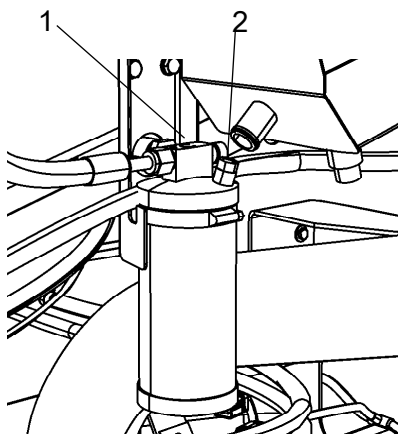
Fig. Filtre de séchage dans le compartiment du moteur 1. Repère vitré 2. Indicateur d'humidité
