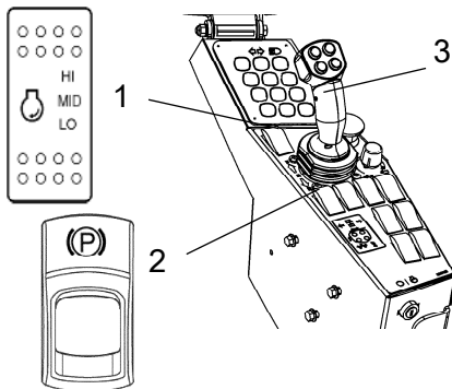
Fig. Tableau de bord 1. Sélecteur de vitesse 2. Frein de stationnement 3. Levier de manœuvre AV/AR
