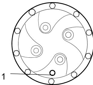
Fig. Réducteur planétaire/position de vidange 1. Bouchon
