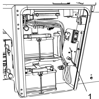
Fig. Cache, côté gauche 1. Interrupteur-sectionneur des batteries
