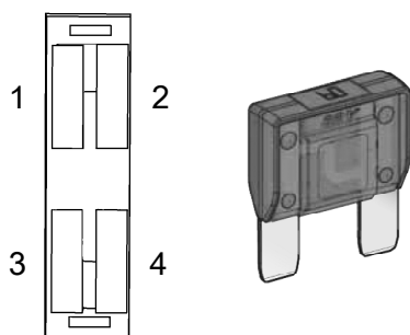
Fig. Boîte à fusibles, interrupteur-sectionneur des batteries
