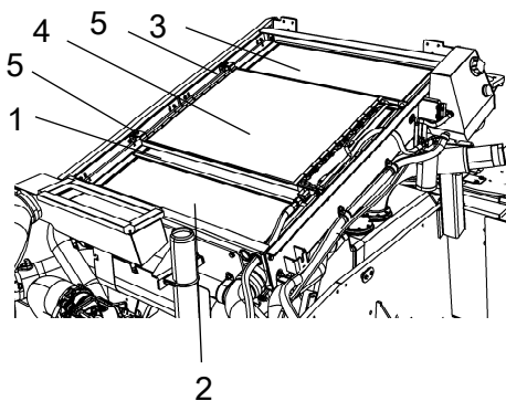
Fig. Compartiment moteur
