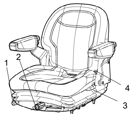
Fig. Siège du conducteur 1. Verrouillage - Réglage longitudinal 2. Réglage du poids 3. Inclinaison du dossier 4. Ceinture
