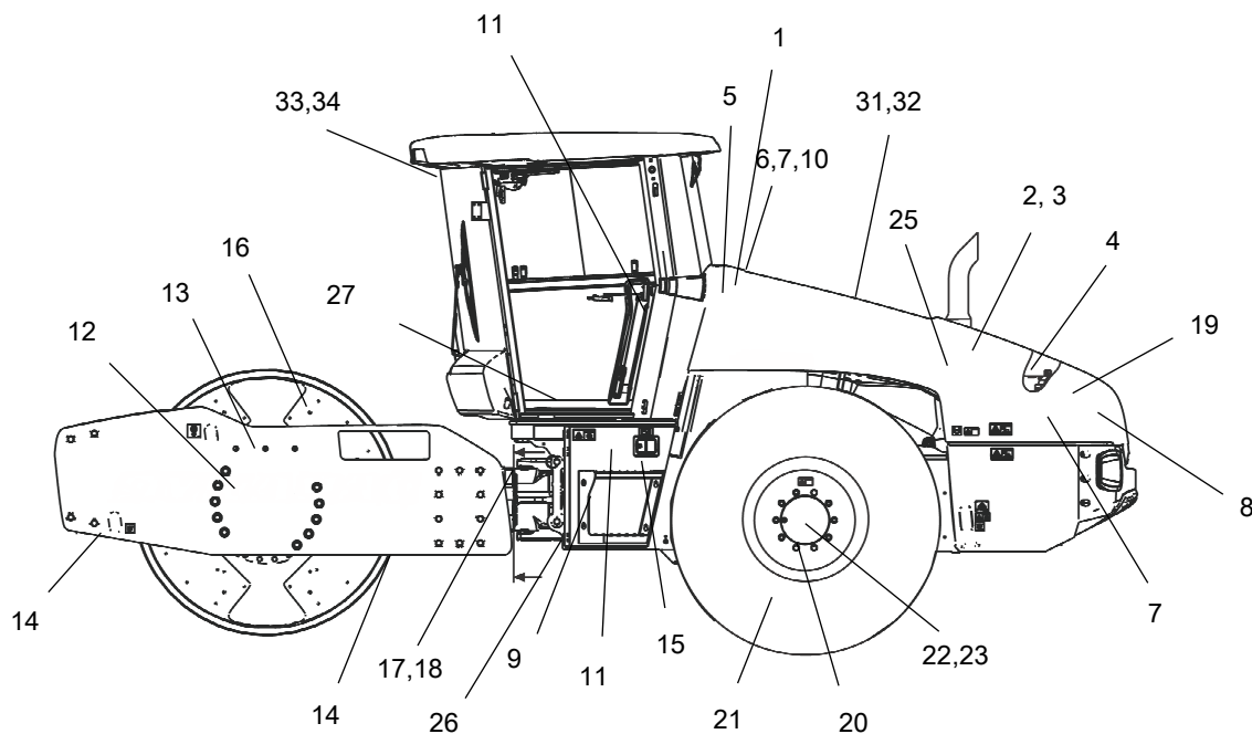
Fig. Points d'entretien et de révision
