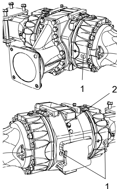
Fig. Contrôle du niveau - logement du différentiel
