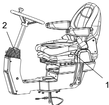
Fig. Poste du conducteur 1. Levier de blocage - rotation 2. Levier de blocage - angle de la colonne de direction
