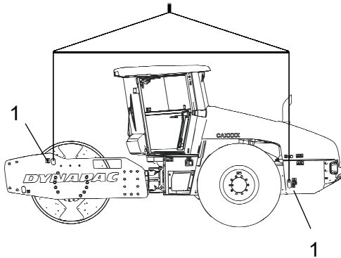
Fig. Rouleau prêt au levage 1. Plaque de levage
