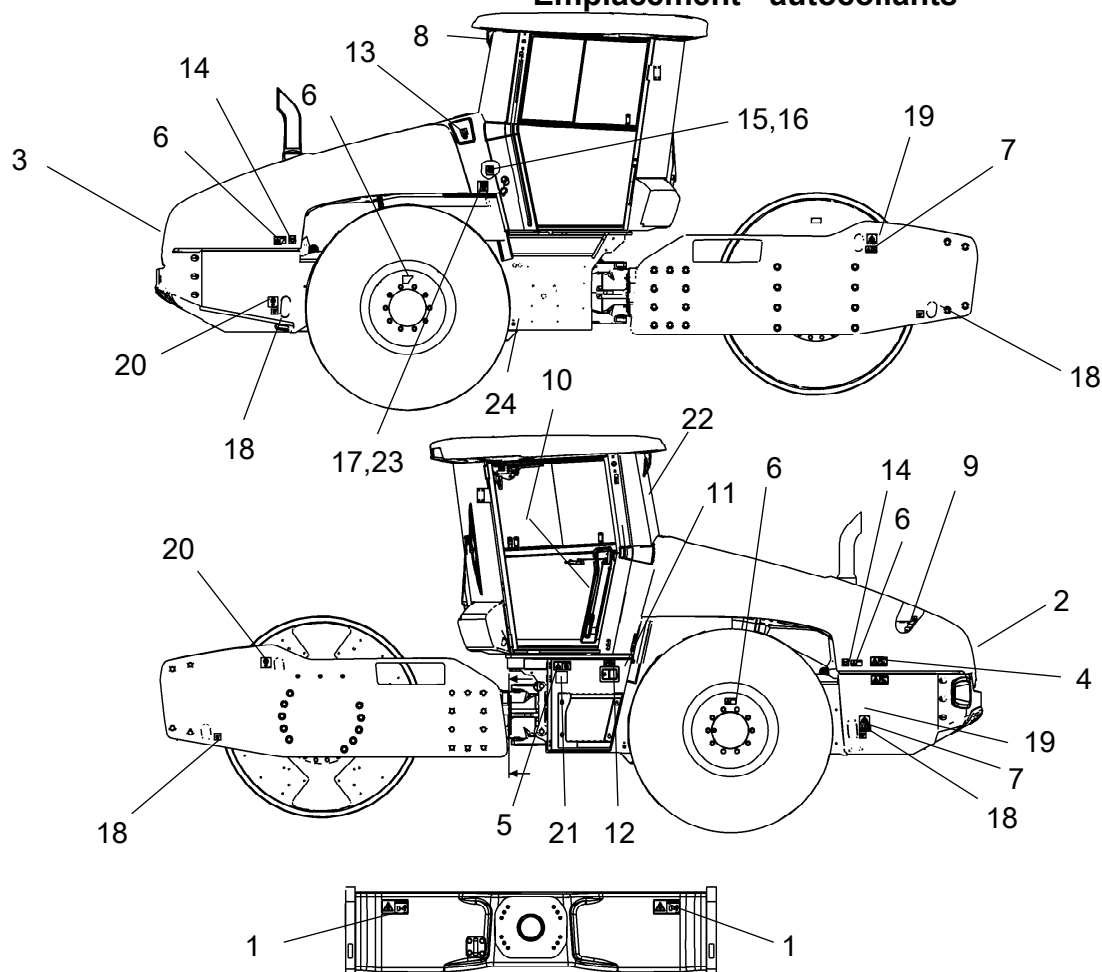
Fig. Emplacement, autocollants et plaques
