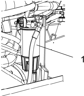
Fig. Compartiment moteur 1. Préfiltre à carburant
