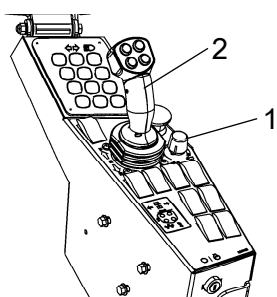
Fig. Tableau de bord 1. Potentiomètre (limiteur de régime) 2. Levier de manoeuvre AV/AR
