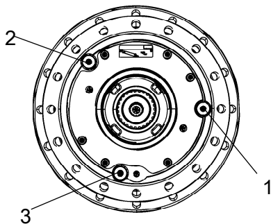
Fig. Contrôle de niveau d'huile - réducteur de cylindre
