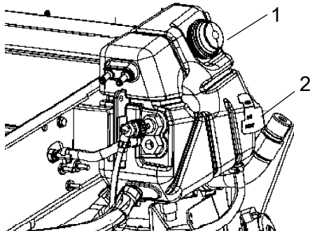
Fig. Réservoir d'expansion 1. Bouchon de remplissage 2. Indicateur de niveau
