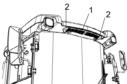
Fig. Cabine 1. Filtre à air neuf (x 2) 2. Vis (x 3)
