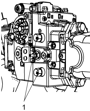
Fig. Pompe de transmission 1. Soupape de dérivation
