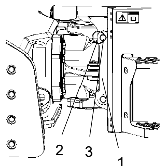
Fig. Verrouillage du joint de direction 1. Bras de verrouillage 2. Goupille d'arrêt 3. Pointe de verrouillage
