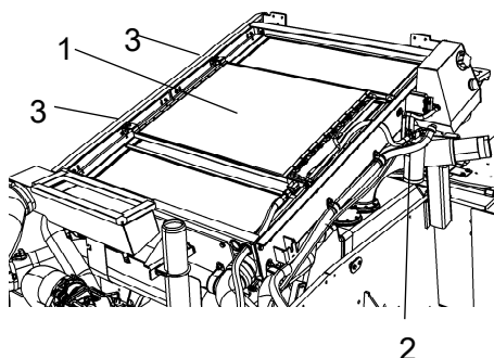
Fig. Compartiment moteur
