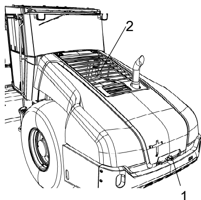
Fig. Capot du moteur 1. Verrou du moteur 2. Grille de protection
