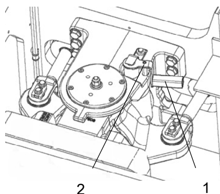
Fig. Verrou articulation centrale, ouverte 1. Poignée de verrouillage 2. Pointe de verrouillage
