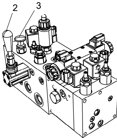
Fig. Distributeur, compartiment moteur 2. Bras de la pompe 3. Bouton de desserrage du frein
