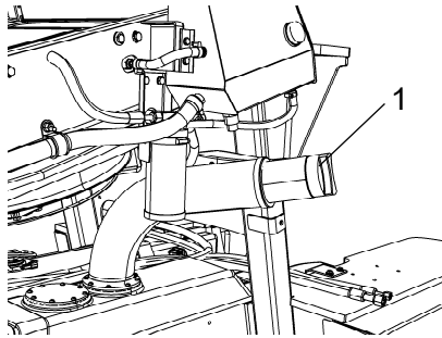
Fig. Réservoir de carburant 1. Tuyau de remplissage
