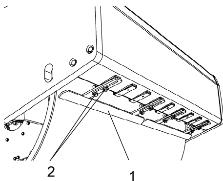
Fig. Racloirs 1. Lame de racleur (x 4) 2. Vis
