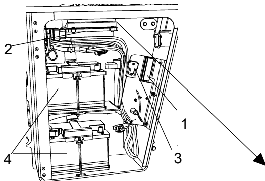
Fig. Cache, côté gauche 1. Boîte à fusibles 2. Unité de commande du moteur (ECM) 3. Fusible 30A, boîtier ECM (IIIB/T4i) Relais 20A, boîtier ECM (IIIA/T3) 4. Batteries x 2 unités)
