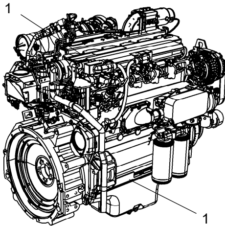
Fig. Moteur 1. Plaque d'identification moteur
