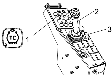
Fig. Tableau de bord 1. Contrôle de la traction (antipatinage) 2. Levier de manœuvre AV/AR 3. Potentiomètre (limiteur de régime)
