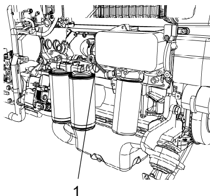
Fig. Compartiment moteur 1. Jauge d'huile
