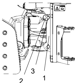
Fig. Verrouillage du joint de direction 1. Bras de verrouillage 2. Goupille d'arrêt 3. Pointe de verrouillage
