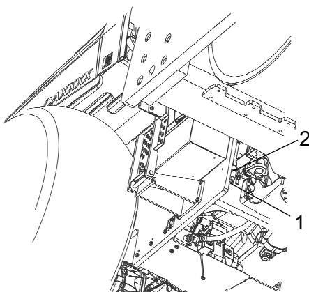
Fig. Dessous droit du rouleau
