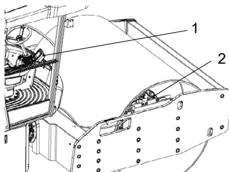
Fig. Composants principaux 1. Écran avec affichage de la valeur CMV 2. Capteur/Unité processeur
