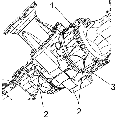
Fig. Essieu arrière, dessous 1. Bouchons de niveau/remplissage (x 3) 2. Bouchons de vidange (x 3) 3. Bouchons de remplissage (x 2)
