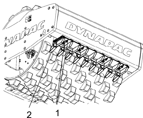
Fig. Raclete 1. Șuruburi 2. Dințe racletă
