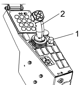
Fig. Tablou de comandă 1. Potentiometru (limitator de viteză) 2. Manetă de direcție înainte/înapoi
