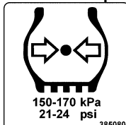
Presiunea pneurilor
