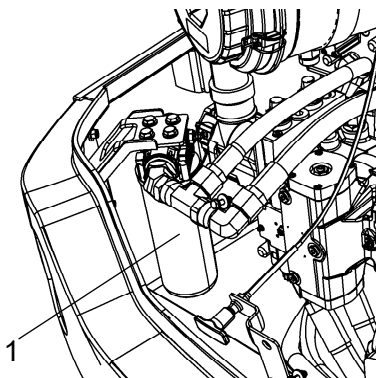
Fig. Compartiment motor 1. Filtru de ulei hidrolic (x 1).
