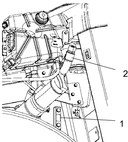
Fig. Rezervor hidraulic 1. Ochi de vizitare 1. Conductă de alimentare
