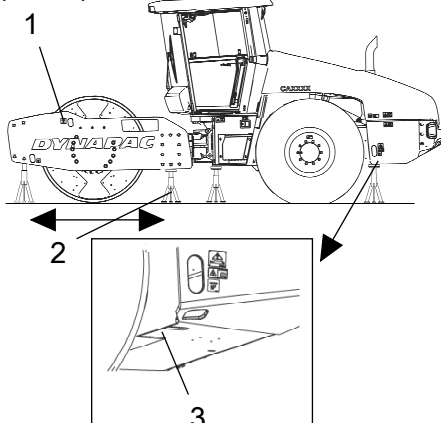
Figura. Vibrocompactor ridicat cu un cric 1. Placa de ridicare 2. Cric 3. Marcaj
