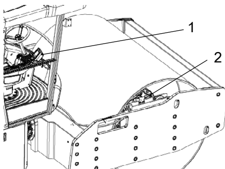
Fig. Componentes principales
