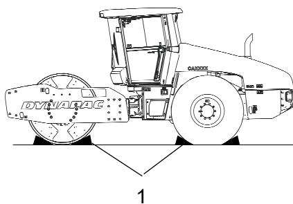
Fig. Colocación 1. Calzos
