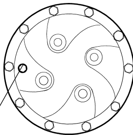
Fig. Planetario / posición de relleno 1. Tapón
