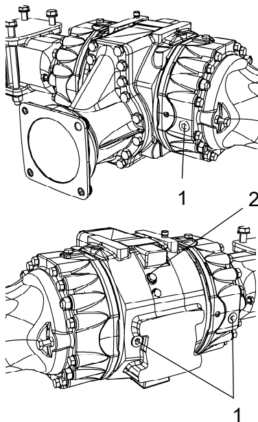
Fig. Control de nivel - caja del diferencial 1. Tapones de nivel (x 3) 2. Tapón de llenado
