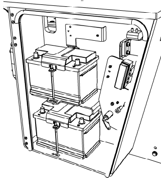
Figura. Baterías
