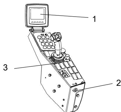
Fig. Panel de control 1. Monitor 2. Llave de arranque 3. Freno de estacionamiento
