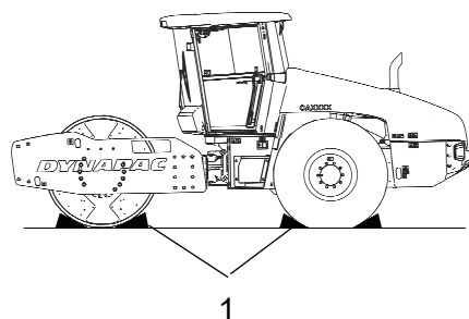
Fig. Colocación 1. Calzos
