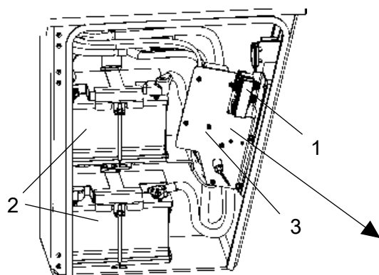
Fig. Cubierta, lado izquierdo
