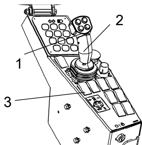
Fig. Panel de control 1. Interruptor, conexión/desconexión de vibraciones 2. Palanca de avance/retroceso 3. Freno de estacionamiento
