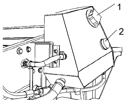
Afb. Expansievat 1. Tankdop 2. Kijkglas
