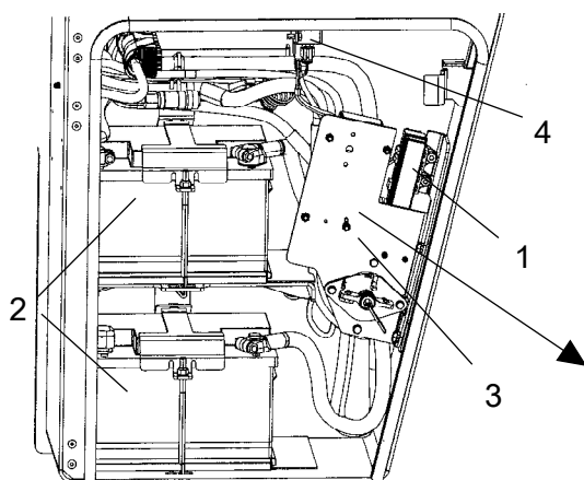
Afb. Klep, linkerzijde 1. Zekeringenkast 2. Accu's (x2) 3. Accuscheiderplaat 4. Voorverwarmingsrelais, 120A
