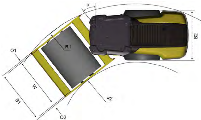
Afmetingen, bovenkant
