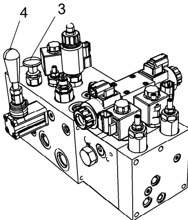
Abb. Ventilblock, Motorraum 3. Bremsfreigabeknopf 4. Pumpenarm
