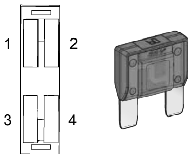
Abb.: Sicherungskasten, Batterietrennschalter
