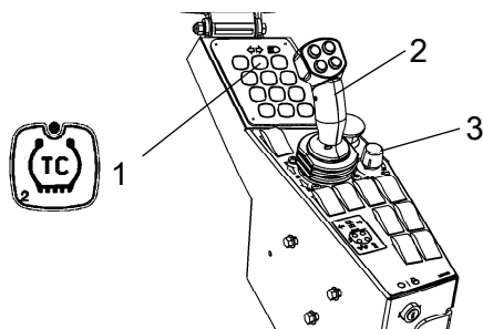
Abb. Bedienkonsole 1. TC (Antischlupfregelung) 2. Vor-/Rückwärtsfahrhebel 3. Potentiometer (Geschwindigkeitsbegrenzer)
