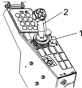
Abb. Bedienkonsole 1. Potentiometer (Geschwindigkeitsbegrenzer) 2. Vor-/Rückwärtsfahrhebel
