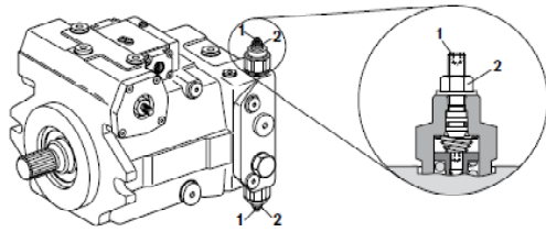
Abb. Antriebspumpe – Überströmventile 1. Schraube 2. Kontermutter
