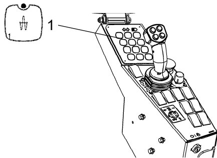
Abb.: Bedienkonsole 1. Große Amplitude
