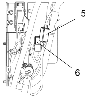
5. Sicherung Motorsteuerung (ECM) (F13), 30 A 6. Kraftstoff-Solenoidrelais
