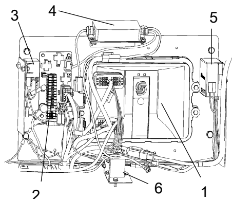
Abb. Hauptschaltkasten
