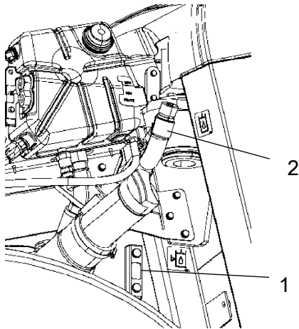
Abb. Hydrauliköltank 1. Schauglas 2. Einfüllstutzen
