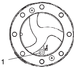
Abb. Planetengetriebe / Stellung zum Ölablassen 1. Schraube
