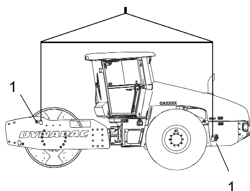
Abb.: Walze zum Anheben vorbereitet 1. Leistungsschild
