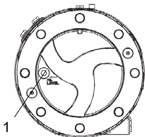
Abb. Planetengetriebe / Stellung zum Ölauffüllen 1. Schraube
