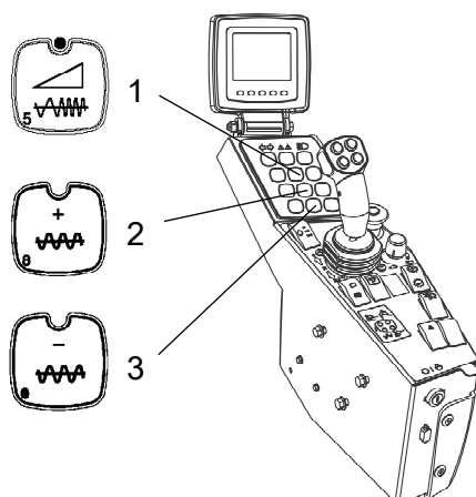
Abb.: Funktionstasten 1. Frequenzregulierung 2. Frequenz erhöhen 3. Frequenz verringern
