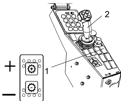
Abb. Bedienkonsole 1. Getriebepositionsschalter 2. Vor-/Rückwärtsfahrhebel
