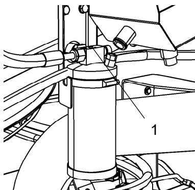
Abb. Trockenfilter 1. Schauglas
