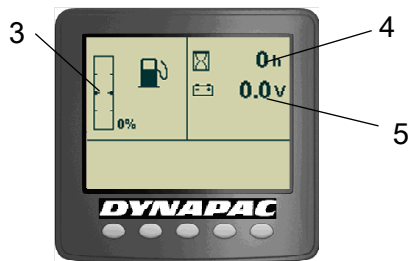
Abb.: Statusbild 3. Kraftstofffüllstand 4. Betriebsstundenzähler 5. Voltmeter
