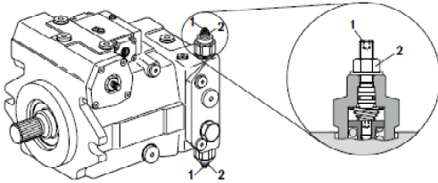
Abb. Antriebspumpe – Überströmventile 1. Schraube 2. Kontermutter
