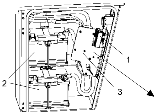
Abb. Abdeckung, linke Seite 1. Sicherungsdose 2. Batterien (x2) 3. Batterietrennschalter-Platte
