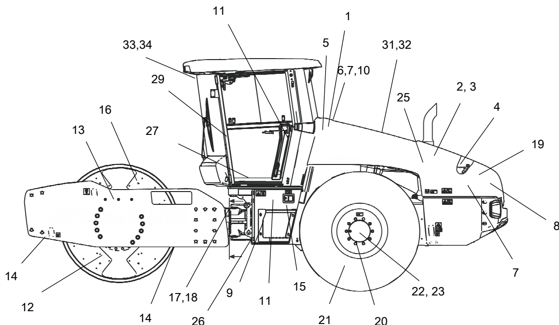
Abb. Service- und Kontrollpunkte
