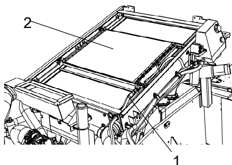
Abb. Klimaanlage 1. Kühlmittelschläuche 2. Kondensatoreinheit
