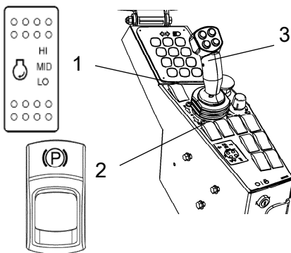
Abb. Bedienkonsole 1. Drehzahlwähler 2. Feststellbremse 3. Vor-/Rückwärtsfahrhebel
