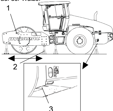
Abb. Mit Wagenheber angehobene Walze
