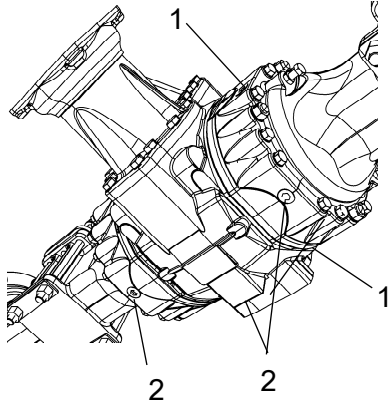
Abb. Hinterachse, Unterseite 1. Ölstand-/Öleinfüllschrauben (x 3) 2. Ablassschrauben (x 3)
