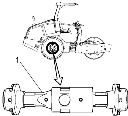
Abb. Ölstandskontrolle - Differentialgehäuse 1. Ölstand/Öleinfüllschraube
