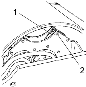
Abb. Bandage, Vibrationsseite 1. Gummielmente 2. Schrauben
