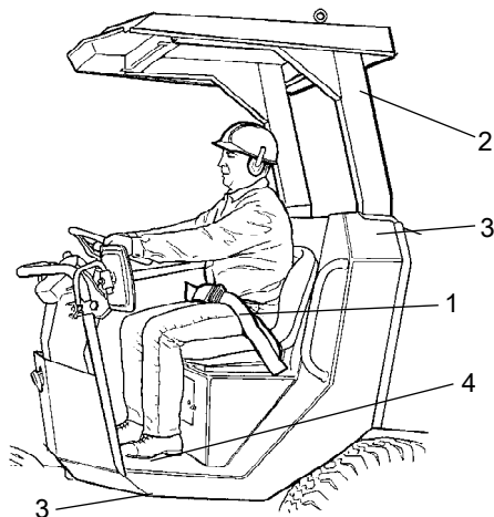
Abb. Fahrersitz
