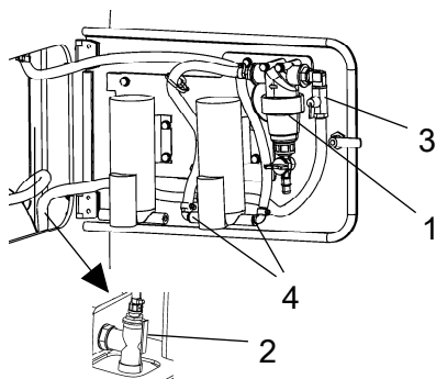
Рис. Насосная система
