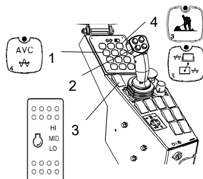
Рис. Панель управления 1. Автоматическая система контроля вибрации (AVC) 2. Переключатель вибрации, вкл./выкл. 3. Переключатель оборотов 4. Рабочий режим
