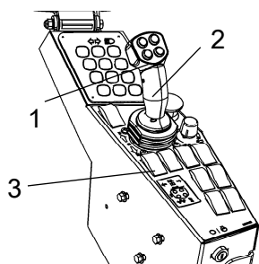
Рис. Панель управления 1. Выключатель вибрации 2. Рычаг прямого/обратного хода 3. Стояночный тормоз
