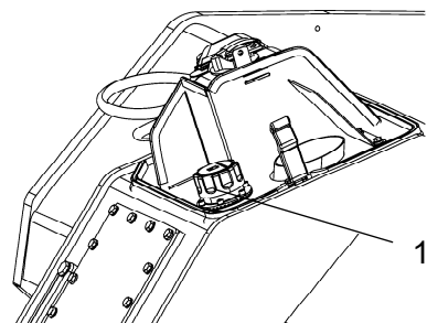
Рис. Задняя рама, левая сторона, спереди 1. Крышка гидравлического бака
