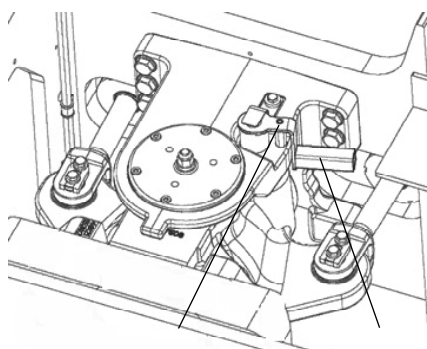
Рис. Блокировка шарнирного сочленения (открыта) 1. Запорная ручка 2. Стопорный штифт
