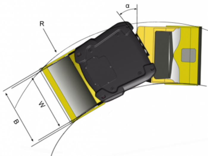
Размеры, вид сверху
