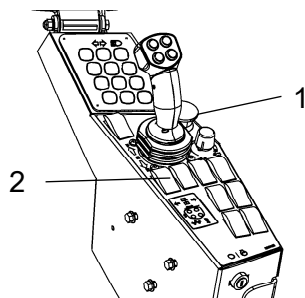
Рис. Панель управления 1. Аварийный останов 2. Стояночный тормоз
