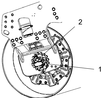
Рис. Проверка уровня масла - передача вальца
