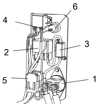
Рис. Главная панель предохранителей 1. Главный выключатель 2. Реле предварительного нагрева (100A) 3. Предохранитель (F20) (125A) 4. Реле стартера (50A) 5. Предохранитель (F13, F10, F11) 6. Розетка на 24 В
