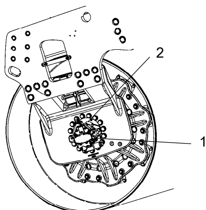
Рис. Проверка уровня масла - передача вальца 1. Пробка уровня 2. Пробка заливного отверстия
