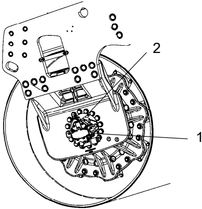
Şekil Yağ seviyesi kontrolü - silindir dişlisi 1. Seviye tapası 2. Doldurma tapası
