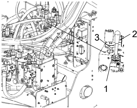
Şekil Fren ayırma valfi 1. Valf 2. Pompa kolu 3. Düğme
