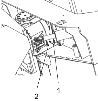
Sekil. Belden kırma kilitli konumda 1. Kamalı pim 2. Kilit
