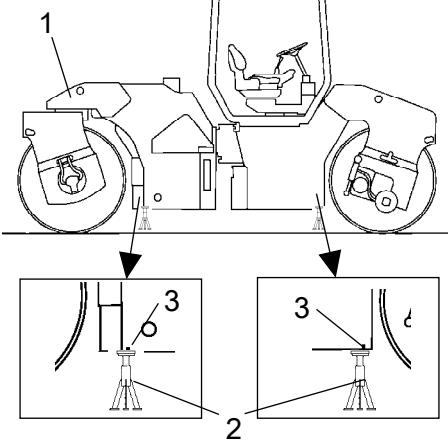
Şekil. Kriko ile kaldırılmış silindir 1. Kaldırma plakası 2. Kriko 3. İşaret
