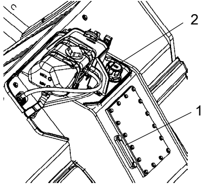
Şekil. Şekil Hidrolik sıvısı deposu 1. Yağ gözetleme camı 2. Doldurma kapağı
