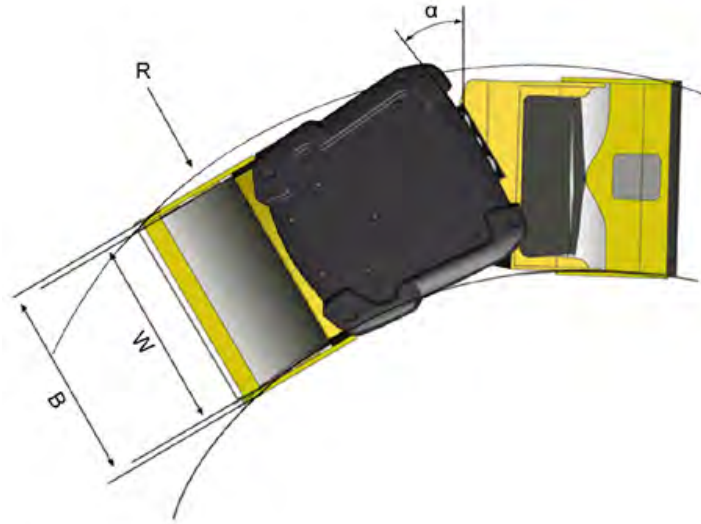
Boyutlar, üstten görünüm
