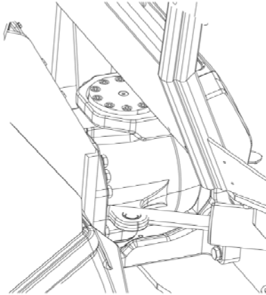
Şekil Direksiyon bağlantısı
