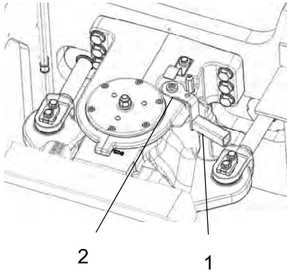
Sekil Direksiyon bağlantısı kilidi, kilitli 1. Kolu kilitleyin 2. Kilitleme saplaması
