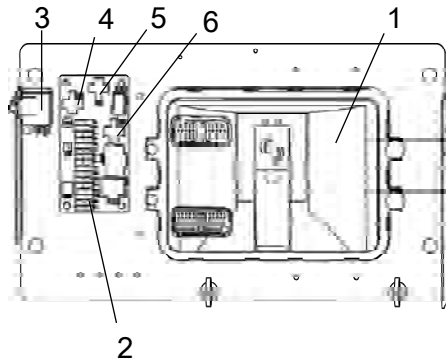
Şekil. Ana sigorta kutusu
