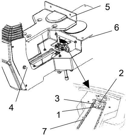
Şekil. Koltuk yatağı 1. Gres nipel 2. Dişli çark 3. Direksiyon zinciri 4. Ayarlama vidası 5. Kapak 6. Kızak rayları 7. İşaretleme
