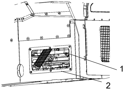
Şekil. Motor bölmesi, sağ taraf 1. Yağ filtresi 2. Servis paneli
