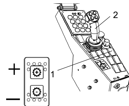
图例：控制面板 1. 齿轮位置开关 2. 前进/后退档杆
