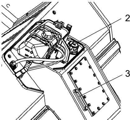
图液压油箱 2. 油箱盖 3. 窥镜
