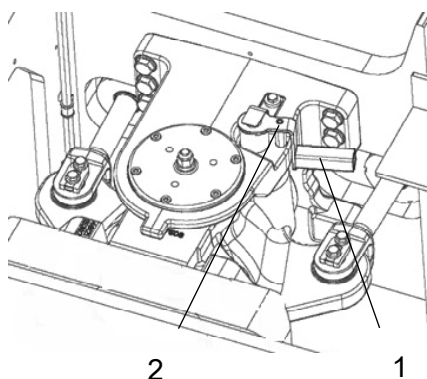
图：转向接头锁闭，打开 1. 锁紧操纵杆 2. 定位销
