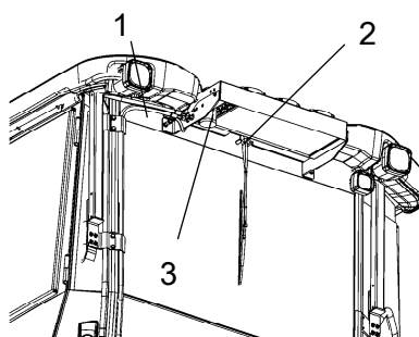
图：空调 1. 制冷剂软管 2. 冷凝器配件 3. 干燥过滤器
