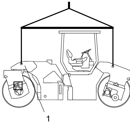
图：待吊装压路机 1. 吊装铭牌
