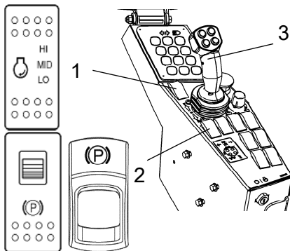
图：控制面板 1. Rpm 开关 2. 驻车制动器 3. 前进/后退档杆
