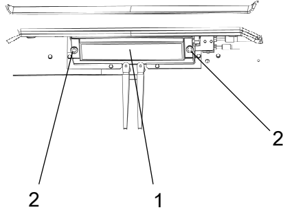
图驾驶室，前侧 1. 空气过滤器 (x1) 2. 螺丝 (x2)
