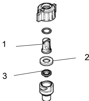
图例：喷嘴 1. 喷嘴 2. 垫圈 3. 过滤器
