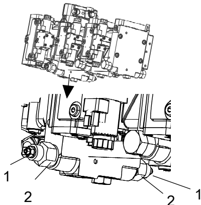
图：推进泵 1. 牵引阀 2. 旁通阀
