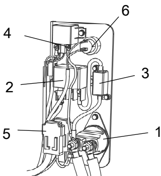
图：主熔断器板 1. 主开关 2. 预热继电器（100 安培） 3. 熔断器（F20）（125 安培） 4. 启动机继电器（50 安培） 5. 熔断器（F13、F10、F11） 6. 电源插座 24 伏
