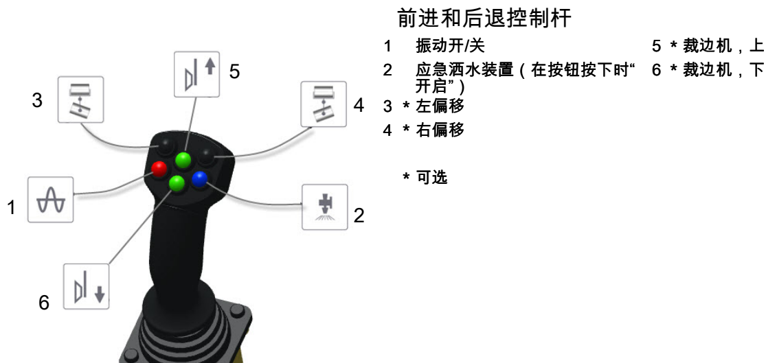
图：前进和后退控制杆
