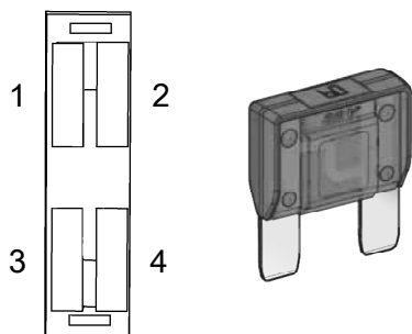
图：熔断器盒，主开关
