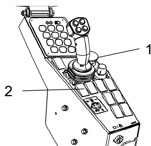
Obr. Ovládací panel 1. Nouzový vypínač 2. Parkovací brzda
