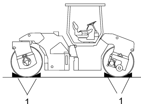
Obr. Umístění 1. Klíny
