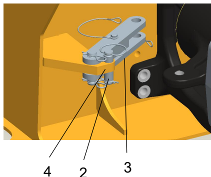
Obr. Spojení v odjištěné poloze 2. Pojistný čep 3. Pojistné rameno 4. Pojistné oko
