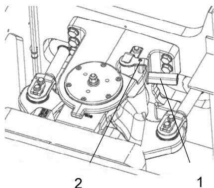
Fig. Blocco dello snodo dello sterzo, aperto 1. Maniglia di blocco 2. Grano di bloccaggio
