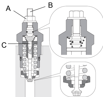
Fig. Valvola di traino
