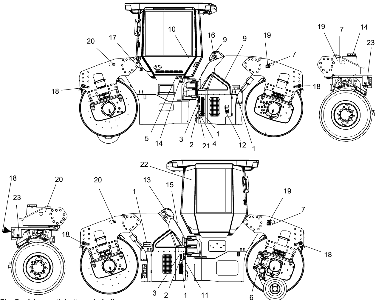
Fig. Posizione, etichette e simboli
