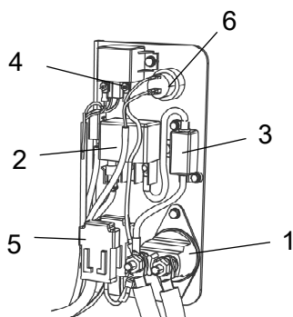
Fig. Quadro fusibili principale 1. Interruttore della batteria 2. Relè di preriscaldamento (100A) 3. Fusibile (F20) (125 A) 4. Relè di avvio (50A) 5. Fusibili (F13, F10, F11) 6. Presa di alimentazione 24 V
