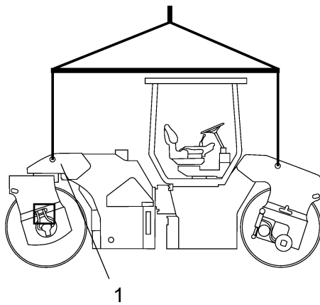
Fig. Rullo preparato per il sollevamento 1. Targhetta per il sollevamento
