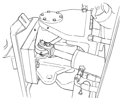
Fig. Snodo dello sterzo
