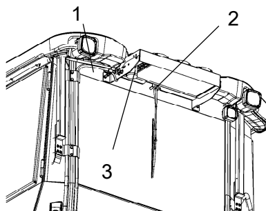
Fig. Aria condizionata 1. Tubi del refrigerante 2. Elemento condensatore 3. Asciugatura del filtro
