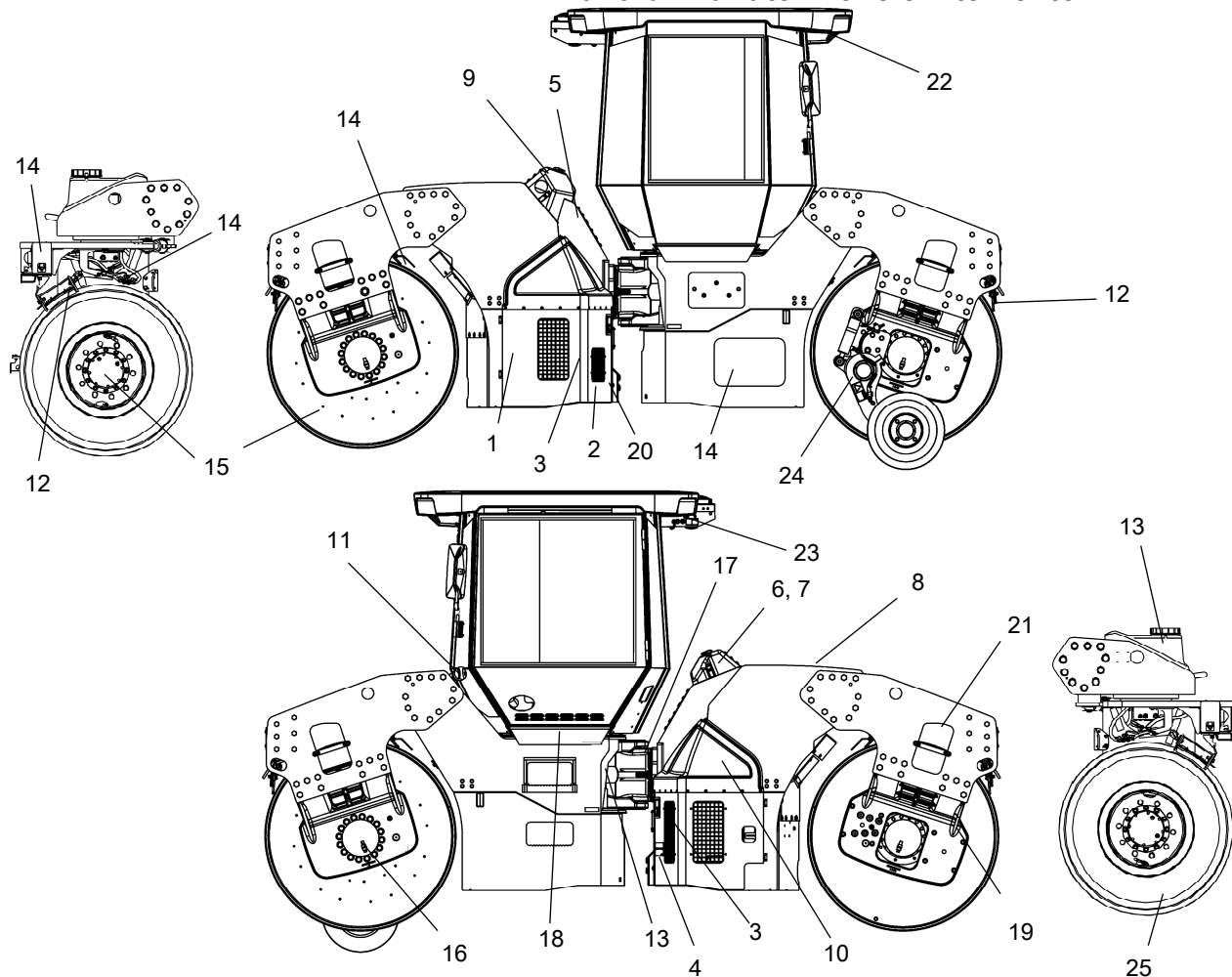
Fig. Punti di manutenzione e intervento
