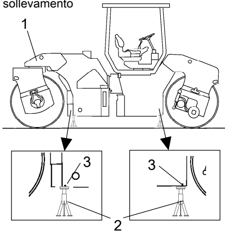
Fig. Rullo alzato con il martinetto 1. Piastra di sollevamento 2. Martinetto 3. Contrassegno
