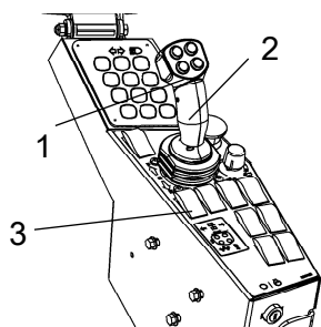
Fig. Quadro di controllo 1. Interruttore di attivazione/disattivazione delle vibrazioni 2. Leva di comando avanti/indietro 3. Freno di stazionamento
