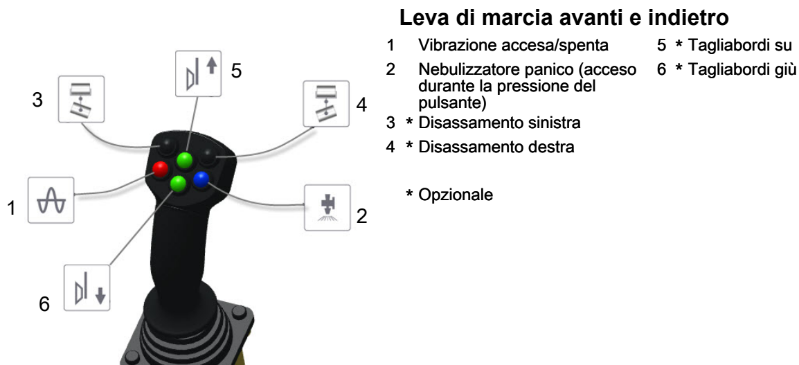
Fig. Leva di marcia avanti e indietro
