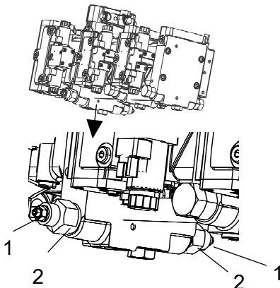
Fig. Pompa di trasmissione 1. Valvola di traino 2. Valvola di by-pass
