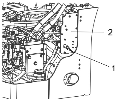
Fig. Vano batteria 1. Interruttore principale 2. Pannello fusibili principali
