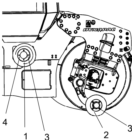
Fig. Sostituzione dell'utensile 1. Compattatore per bordi 2. Tagliabordi 3. Giunto a vite 4. Pomello per volante tagliabordi/compattatore
