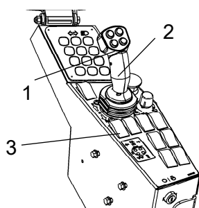
Fig. Quadro di controllo
