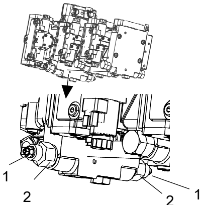
Fig. Pompa di trasmissione 1. Valvola di traino 2. Valvola di by-pass
