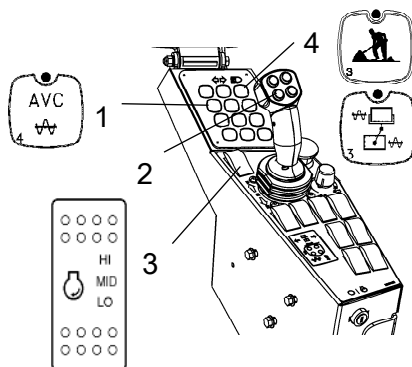
Fig. Quadro di controllo 1. Controllo automatico delle vibrazioni (AVC) 2. Interruttore delle vibrazioni ON/OFF 3. Selettore giri/min. 4. Modalità di lavoro
