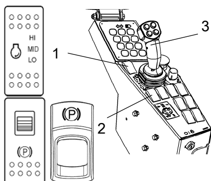
Рис. Панель управления
