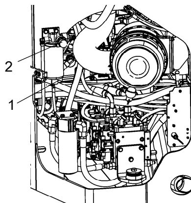
Рисунок. Топливный фильтр 1. Спускная заглушка 2. Ручной насос
