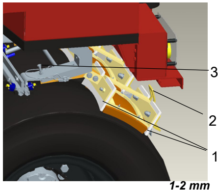
Fig. Rascadores de ruedas 1. Hojas del rascador 2. Gancho de bloqueo 3. Tornillo de ajuste
