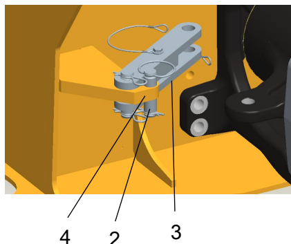
Fig. Articulación desbloqueada
