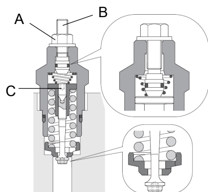
Figura. Válvula de remolque
