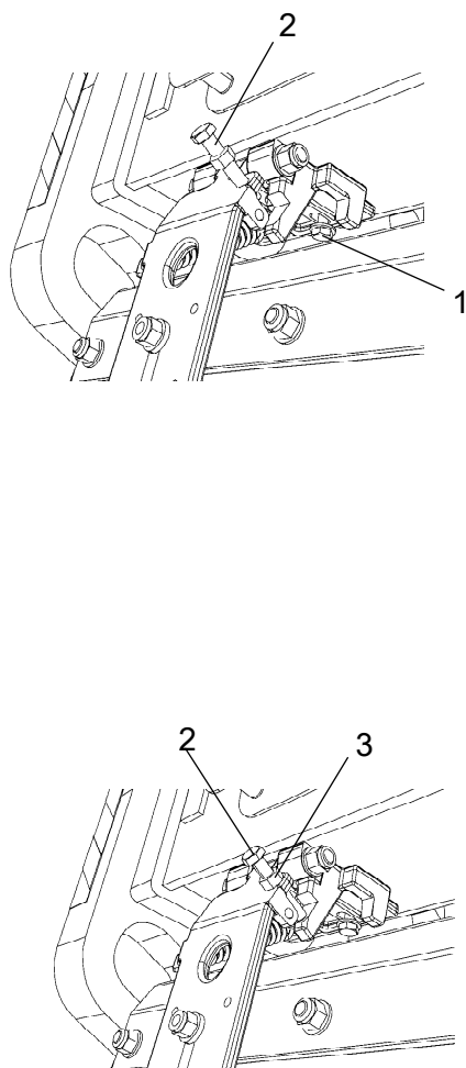
Figura. Ajuste del rascador 1. Unidad de retención 2. Tornillo de ajuste 3. Contratuerca
