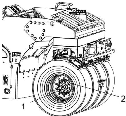
Fig. Comprobación del nivel de aceite - Engranaje de las ruedas 1. Tapón de nivel 2. Tapón de llenado
