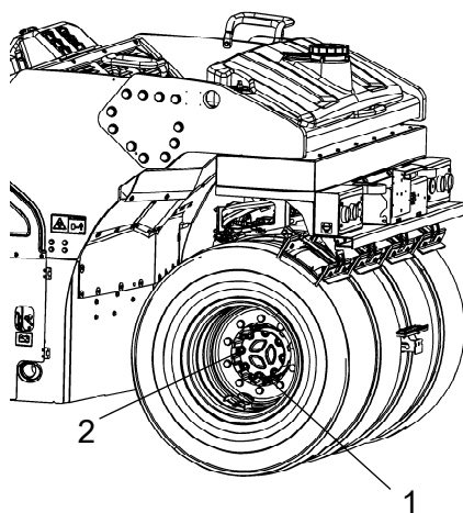
Fig. Engranaje de las ruedas 1. Tapón de drenaje 2. Tapón de ventilación
