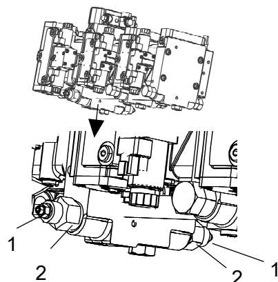
Fig. Bomba de propulsión 1. Válvula de remolque 2. Válvula de bypass
