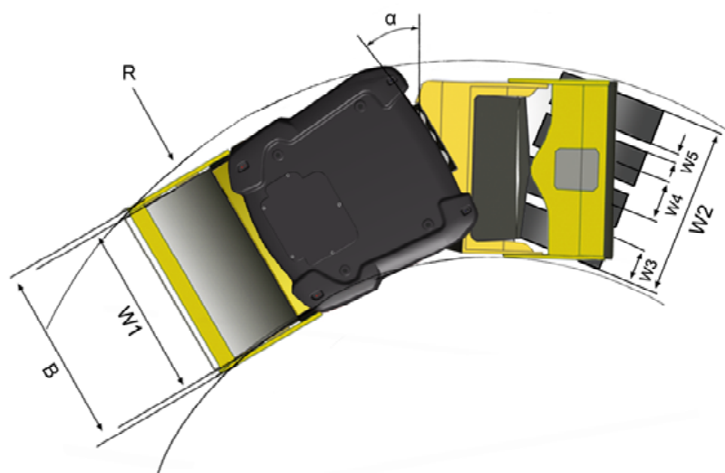
Dimensiones, vista superior
