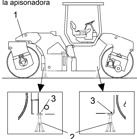
Figura. Apisonadora elevada con un gato
