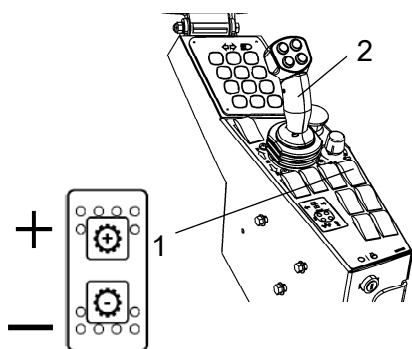
Fig. Panel de control 1. Interruptor de posición de marcha 2. Palanca de avance/retroceso
