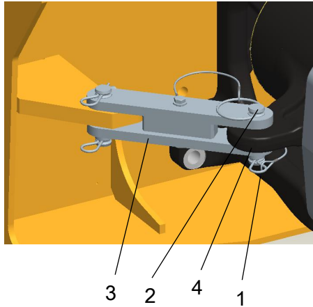
Fig. Articulación en posición bloqueada
