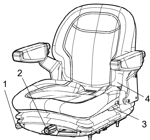
Obr. Sedačka řidiče 1. Stavěcí páčka – nastavení délky 2. Nastavení hmotnosti 3. Úhel opory zad 4. Bezpečnostní pás
