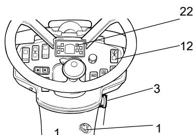
Obrázek. Panel přístrojů 1. Startovací přepínač 3. Nouzové zastavení/rezervní brzda 12. Přepínač, klopení 22. Výstražný panel
