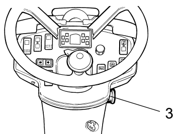
Obr. Ovládací panel 3. Nouzové zastavení/rezervní brzda
