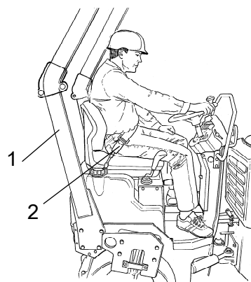
Obr. Poloha sedačky 1. ROPS 2. Bezpečnostní pás
