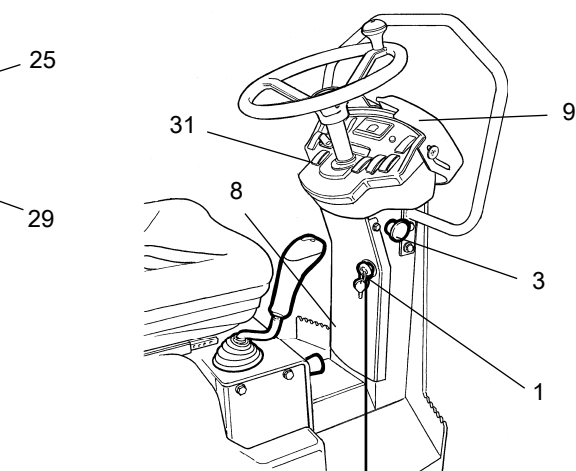
Obr. Stanoviště obsluhy
