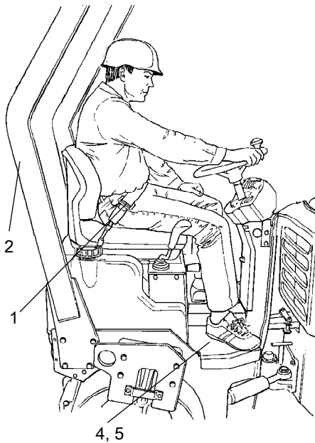
Fig. Chauffeurspositie 1. Veiligheidsgordel 2. Inklapbare rolkooi 4. Rubberen element 5. Anti-slipbescherming
