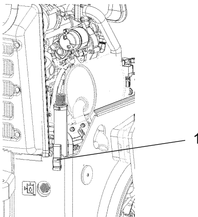
Fig. Motorruimte, rechterkant 1. Kijkglas
