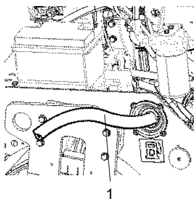
Fig. Brandstoftank
