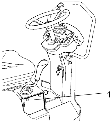
Fig. Vooruit/achteruit-hendel 1. Plaat
