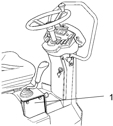
Fig. Vooruit/achteruit-hendel 1. Plaat
