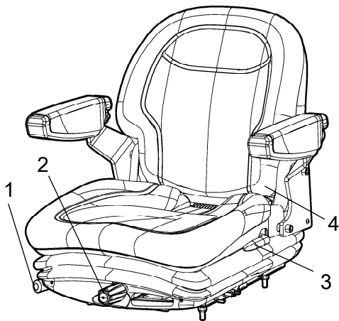
Fig. Förrarstol 1. Låsspak - Längdinställning 2. Viktinställning 3. Ryggstödslutning 4. Sitsbälte
