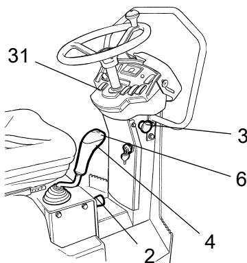
Fig. Reglagepanel 2. Varvtalsreglage 3. Nödstop 4. Vibration Till/från 6. Fram/backreglage 31. Parkeringsbroms
