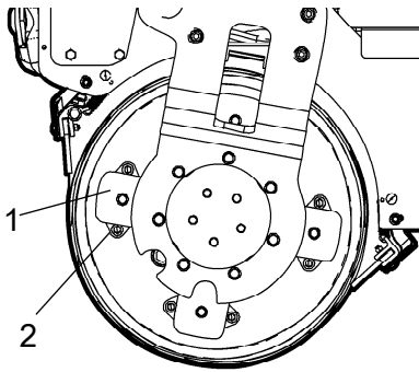
Fig. Valsupphängning 1. Gummiement 2. Fästskruvar
