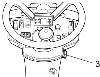
Fig. Reglagepanel 3. Nödstopp
