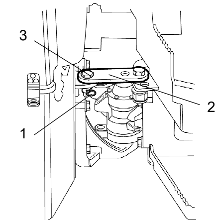
Fig. Styrled 1. Låssprint 2. Låsarm 3. Låsbult
