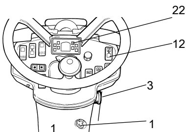
Fig. Instrumentpanel 1. Startströmställare 3. Nödstopp 12. Strömställare bevattning 22. Varningspanel
