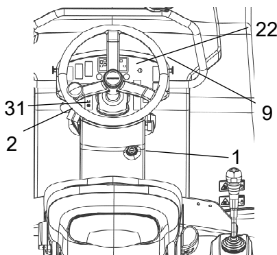
Fig. Pannello strumenti 1. Interruttore di avviamento 2. Comando dell'acceleratore 9. Coperchio strumenti 22. Quadro delle spie 31. Freno di parcheggio
