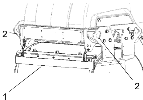
Fig. Raschietti elastici 1. Lama del raschietto 2. Viti di regolazione
