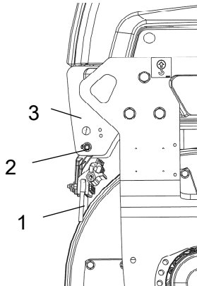
Fig. Tamburo 1. Lama del raschietto 2. Viti di regolazione 3. Piastra di montaggio
