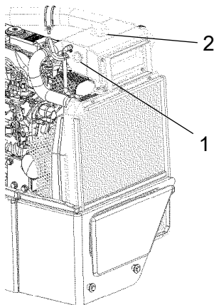
Fig. Recipiente del sistema refrigerante 1. Tappo del serbatoio 2. Contrassegno di livello
