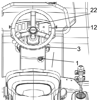
Fig. Pannello strumenti 1. Interruttore di avviamento 3. Arresto di emergenza 12. Interruttore irrorazione 22. Quadro delle spie
