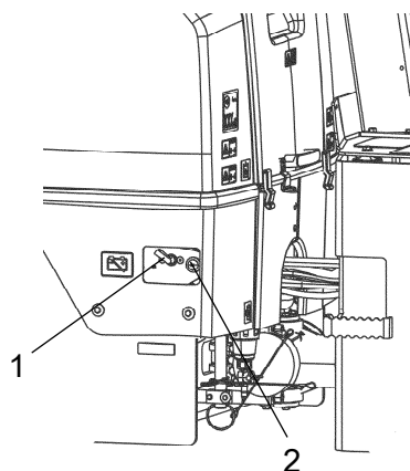
Fig. Vano batteria 1. Sezionatore batteria 2. Presa di alimentazione, 12 V
