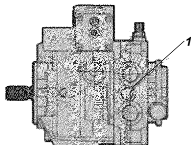
Fig. Pompa di trasmissione - Versione CC 1. Vite di by-pass
