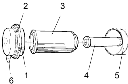
Fig. Filtrul de aer
