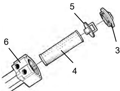
Fig. Filtrul de ulei hidraulic 3. Bușonul
