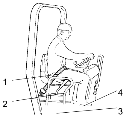
Rys. Siedzenie operatora 1. Pas bezpieczeństwa 2. Poręcz zabezpieczająca 3. Element gumowy 4. Warstwa przeciwpoślizgowa
