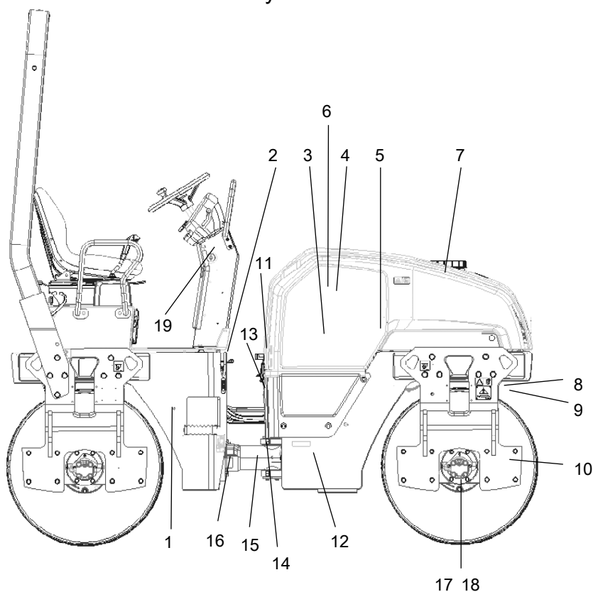
Рис. Позиции проведения технического обслуживания
