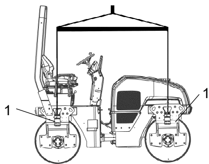
Рис. Подъем катка 1. Подъемная плита
