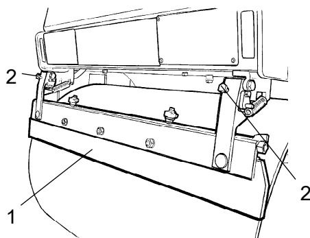
Рис. Подпружиненные скребки 1. Лезвие скребка 2. Регулировочные винты
