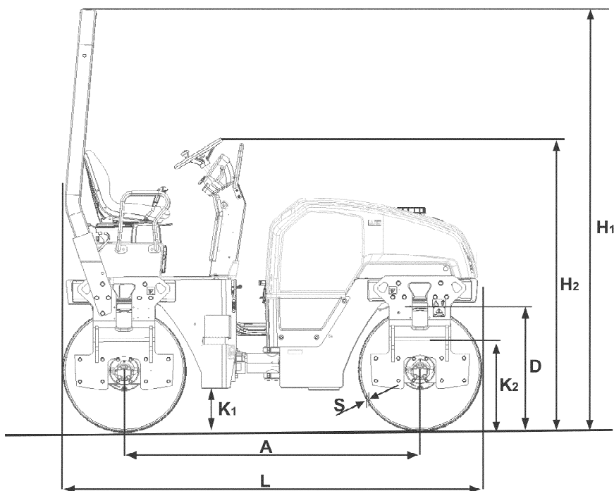
Размеры, вид сбоку
