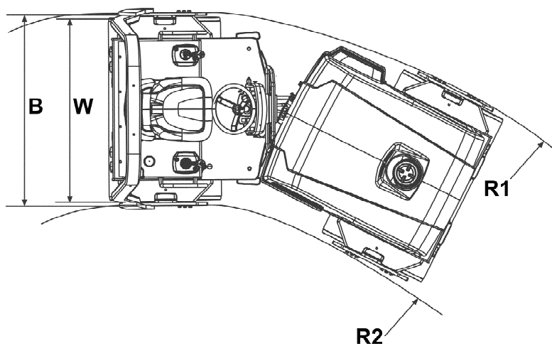
Размеры, вид сверху
