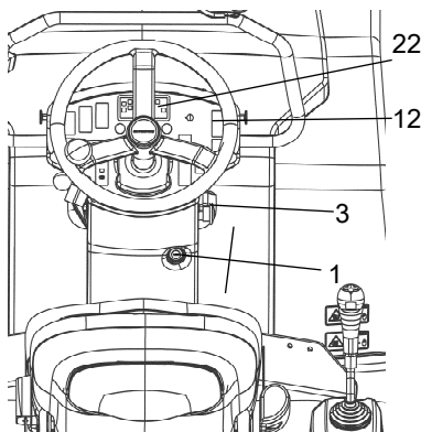
Рис. Приборная панель
