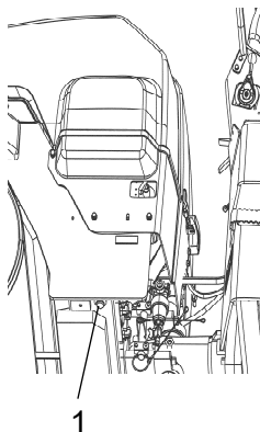
Рис. Левая сторона каркаса 1. Пробка сливного отверстия
