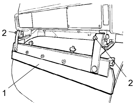
Рис. Подпружиненные скребки 1. Лезвие скребка 2. Регулировочные винты
