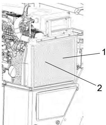
Рис. Отсек двигателя 1. Первый Охладитель воды 2. Радиатор гидравлической жидкости
