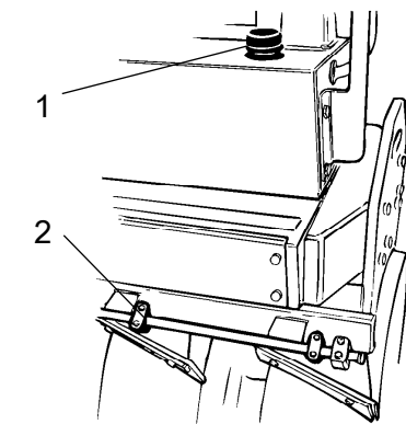
图：车轮支架 1. 加油盖 2. 喷嘴（每个轮胎一个）
