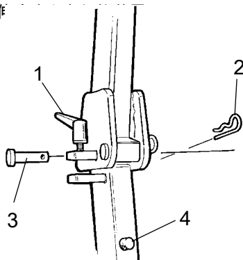
图-翻车保护装置锁定部件 1. 张力螺丝 2. 销子 3. 螺栓 4. 缓冲胶
