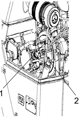
图-发动机室 1 前进/后退档杆 2. 液压油箱盖
