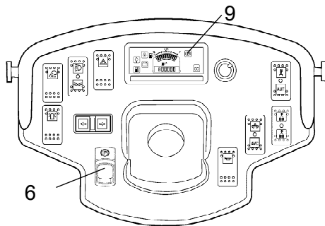
图：仪表板 6. 驻车制动 9. 制动警示灯
