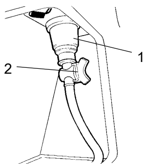
图：左侧踏板 1. 过滤器外壳 2. 截止阀
