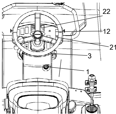
图： 仪表面板 1. 启动开关 3. 紧急停车 12. 开关，洒水 21. 开关，给车轮洒水 22. 警告面板
