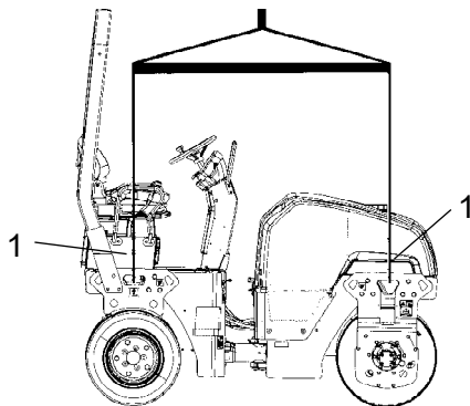
图-起吊压路机 1. 起重铭牌
