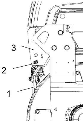
图-钢轮 1. 刮板刀片 2. 调整螺丝 3. 安装板
