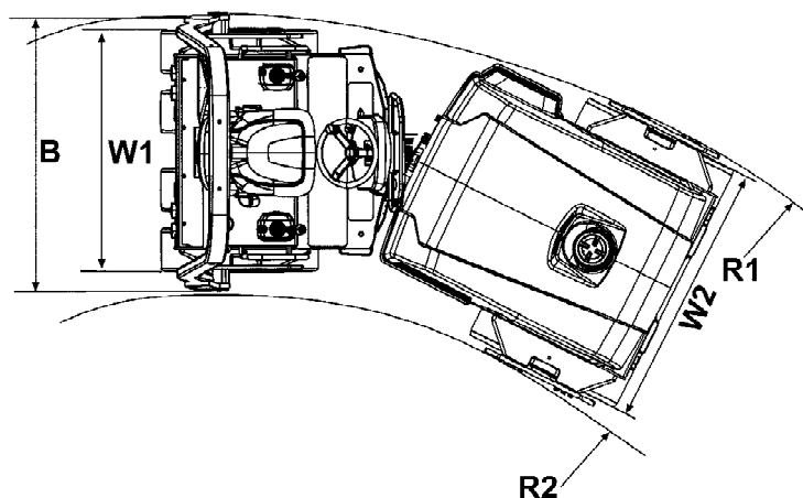
尺寸 - 俯视图
