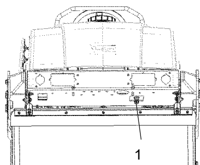
Fig. Vattentank 1. Avtappningsplugg
