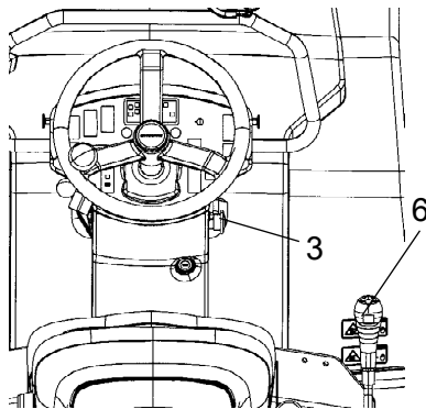
Fig. Reglagepanel 3. Nödstopp 6. Fram/backreglage
