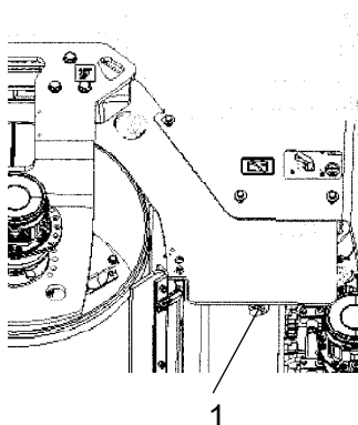
Fig. Vänster ramsida 1. Avtappningsplugg
