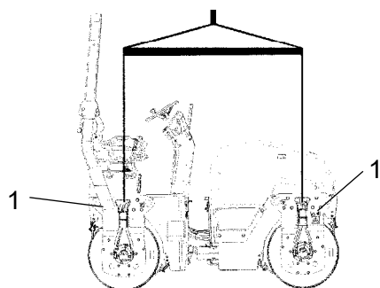
Fig. Lyftning av vält 1. Lyftskylt
