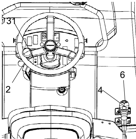
Fig. Reglagepanel 2. Varvtalsreglage 4. Vibration Till/från 6. Fram/backreglage 31. Parkeringsbroms
