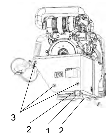
Fig. Motorrum 1. Förfilter 2. Slangklämmor 3. Bultar
