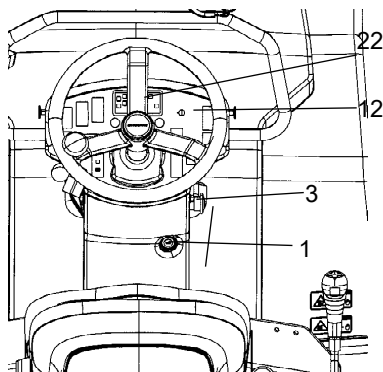
Fig. Instrumentpanel 1. Startströmställare 3. Nödstopp 12. Strömställare bevakning 22. Varningspanel
