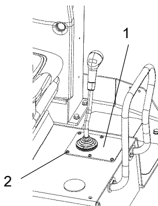
Fig. Fram-/backreglage 1. Skyddsplåt 2. Fästsruvar
