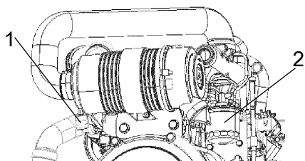
Fig. Luftrenare 1. Indikator 2. Huvudfilter
