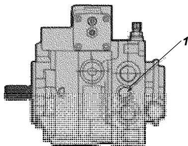
Fig. Framdrivningspump 1. By-pass skruv
