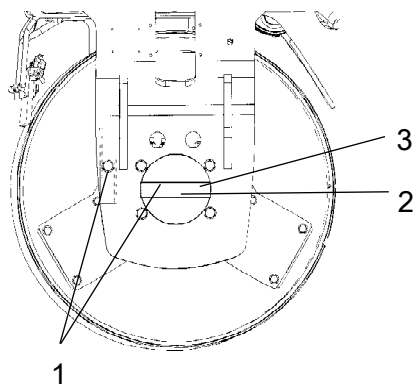
Fig. Vänster valssida
