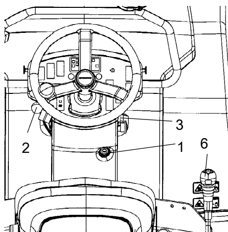
Fig. Instrumentpanel 1. Startströmställare 2. Varvtalsreglage 3. Nödstop 6. Fram/backreglage
