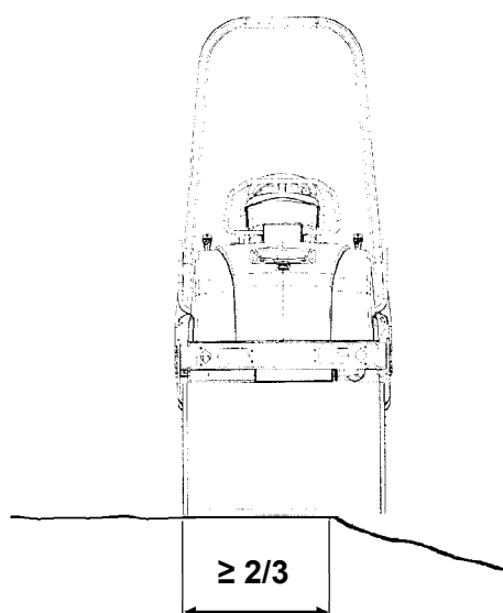
Fig. Valsplacering vid kantkörning
