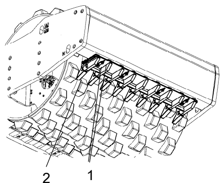
Fig. Raclete 1. Șuruburi 2. Dințe racletă
