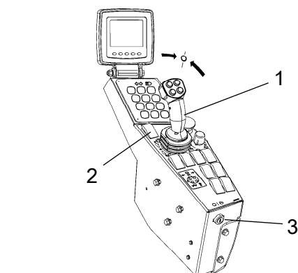
Fig. Tablou de comandă 1. Maneta de deplasare înainte/înapoi 2. Comutator de turație 3. Cheie de contact
