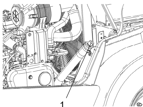
Fig. Réservoir hydraulique 1. Bouchon de remplissage / Filtre d'aération
