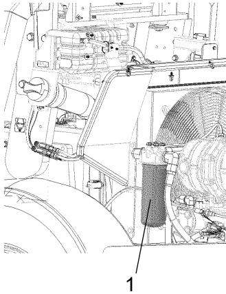
Fig. Compartiment moteur 1. Filtre du fluide hydraulique (1 pièce).
