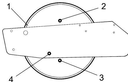
Fig. Cylindre, côté gauche 1. Rainure 2. Bouchon de remplissage 3. Bouchon de vidange/Bouchon magnétique 4. Bouchon de niveau
