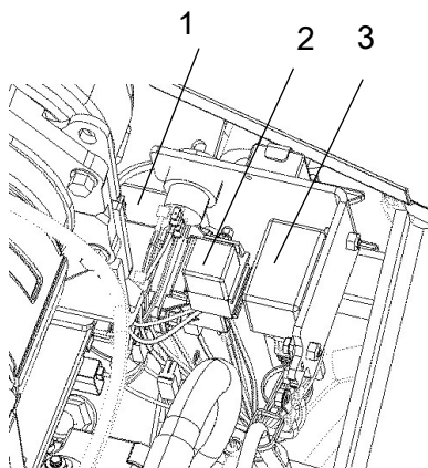
Fig. Relais du compartiment moteur
