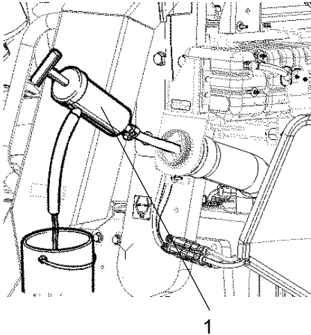
Fig. Réservoir de carburant 1. Pompe de drainage d'huile
