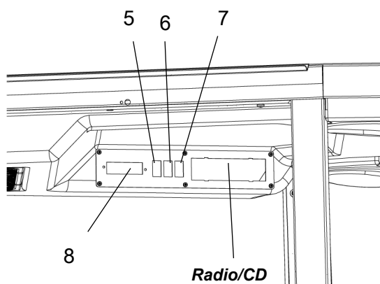
Fig. Toit de la cabine, côté droit
