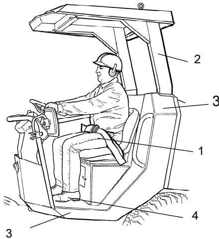
Fig. Poste du conducteur 1. Ceinture de sécurité 2. Structure ROPS 3. Plots élastiques 4. Antidérapant
