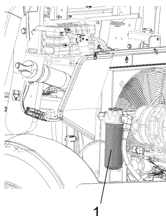
Fig. Compartiment moteur 1. Filtre du fluide hydraulique (1 pièce).
