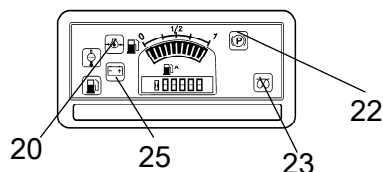
Fig. Panneau de commande 25. Témoin de charge 20. Témoin de pression d'huile 22. Témoin de freinage 23. Voyant de la bougie de préchauffage
