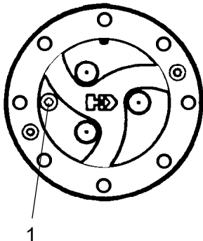
Fig. Réducteur planétaire / position de remplissage 1. Bouchon
