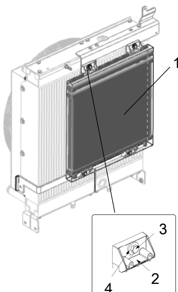
Fig. Condensateur 1. Élément de condensateur 2. Supports (4 unités) 3. Vis (4 unités) 4. Rondelles (4 unités)
