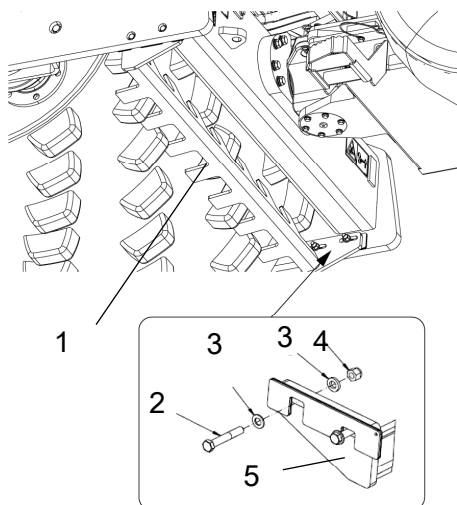
Fig. Racleur (CA1300 PD)
