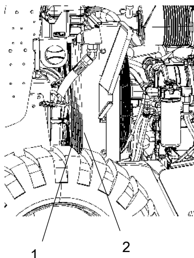
Fig. Compartiment moteur 1. Refroidisseur à eau 2. Refroidisseur du liquide hydraulique
