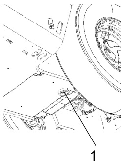
Fig. Réservoir hydraulique, fond 1. Bouchon de vidange
