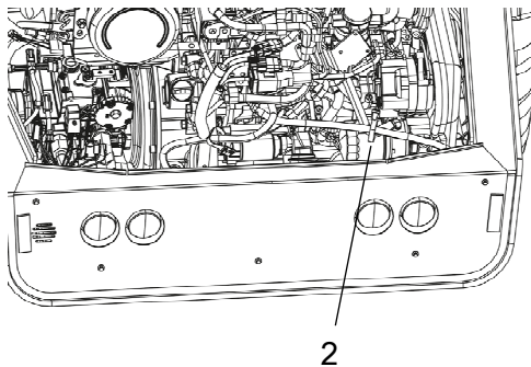
Fig. Compartiment moteur 2. Filtre à huile
