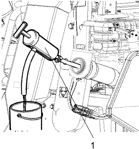
Fig. Réservoir de carburant 1. Pompe de drainage d'huile
