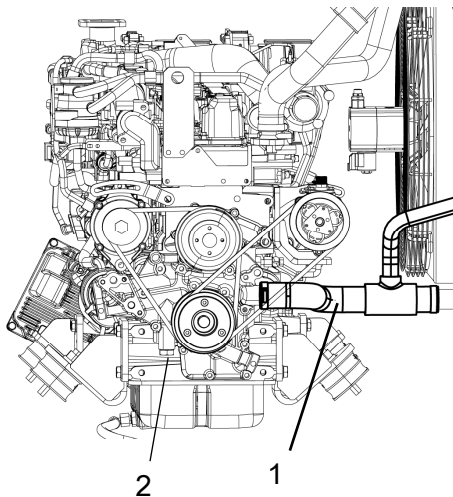
Fig. Vidange, radiateur 1. Tuyau de radiateur 2. Bouchon de vidange (27 mm)
