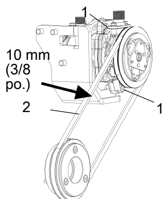
Fig. Compresseur
