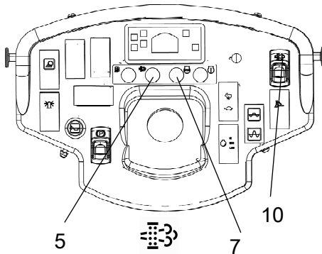
Fig. Pupitre de commande 7. Témoin d'anomalie majeure 5. Témoin de la régénération en stationnement 10. Interrupteur pour la régénération en stationnement du FàPD
