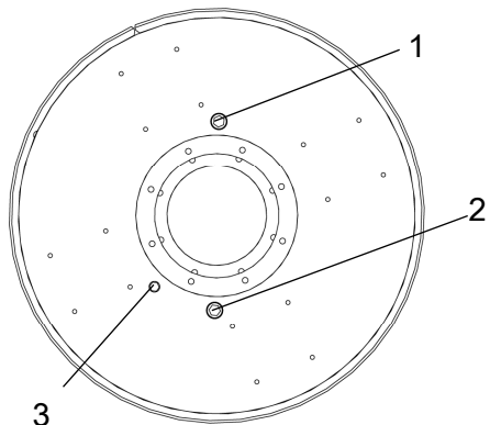
Fig. Rouleau, côté gauche 1. Bouchon de remplissage 2. Bouchon de vidange / Bouchon magnétique 3. Bouchon de niveau
