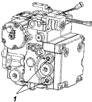
Fig. Pompe de propulsion 1. Soupape de dérivation
