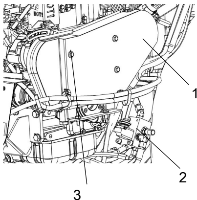
Fig. La salle des machines 1. Protège-courroie 2. Pompe à main 3. Vis
