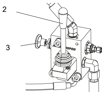
Fig. Pompe de désengagement du frein 2. Bras de la pompe 3. Bouton de desserrage du frein
