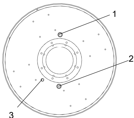
Fig. Rouleau, côté gauche 1. Bouchon de remplissage 2. Bouchon de vidange / Bouchon magnétique 3. Bouchon de niveau
