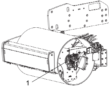
Fig. Remplacement de l'huile - engrenage du cylindre 1. Engrenage du cylindre
