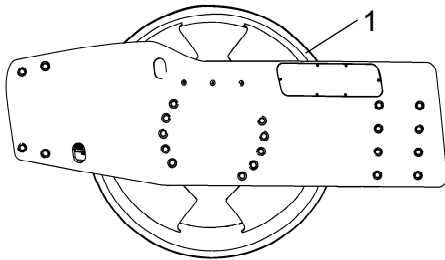
Fig. Côté gauche du cylindre 1. Rainure
