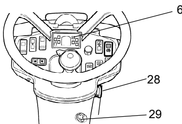
Fig. Tableau de bord 29. Interrupteur de démarrage 28. Arrêt d'urgence 6. Panneau d'avertissement
