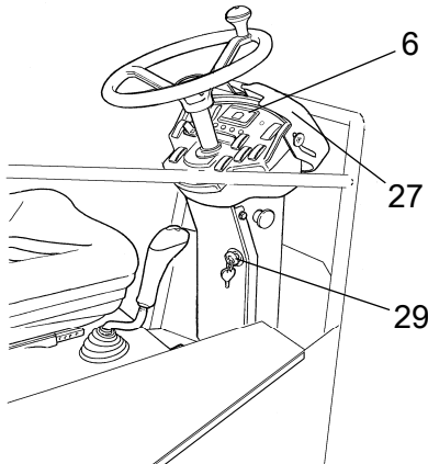
Fig. Tableau de bord 29. Commutateur de démarrage 27. Cache de protection des instruments 6. Panneau pour témoins d'avertissement
