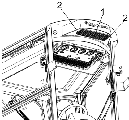
Fig. Cabine 1. Filtre d'air neuf (x 1) 2. Vis (x 8)
