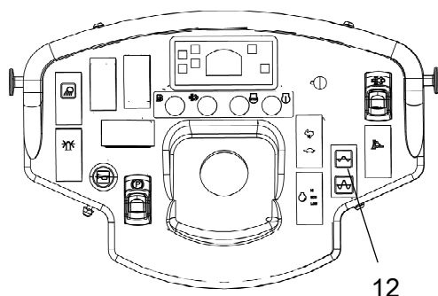
Fig. Tableau de bord 12. Interrupteur de vibrations.
