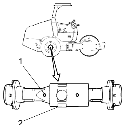
Fig. Essieu arrière 1. Bouchon de niveau/remplissage 2. Bouchon de vidange
