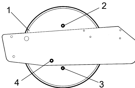
Fig. Cylindre, côté gauche 1. Rainure 2. Bouchon de remplissage 3. Bouchon de vidange / Bouchon magnétique 4. Bouchon de niveau
