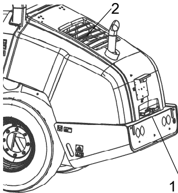
Fig. Capot du moteur 1. Verrou du moteur 2. Grille de protection
