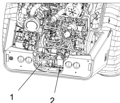
Fig. Compartiment moteur 1. Filtre à carburant 2. Préfiltre à carburant
