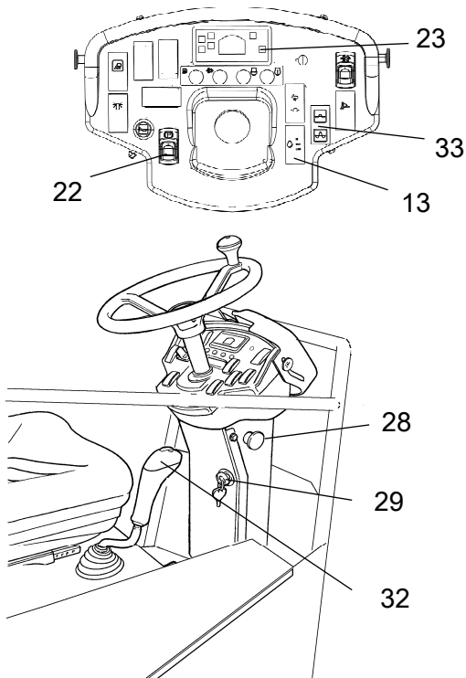
Fig. Pupitre de commande 29. Interrupteur de démarrage 13. Contrôle du régime moteur 28. Arrêt d'urgence 32. Levier de manœuvre AV/AR 33. Commutateur de vibration 23. Témoin de préchauffage 22. Frein de stationnement
