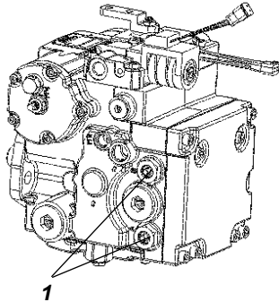
Fig. Pompe de propulsion 1. Soupape de dérivation
