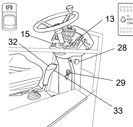
Fig. Tableau de bord 29. Clé 13. Contrôle du régime moteur 28. Arrêt d'urgence 33. Vibration Marche/Arrêt 32. Levier de manoeuvre AV/AR 15. Frein de stationnement
