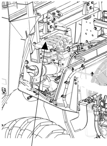
Fig. Réservoir d'eau de refroidissement 1. Bouchon de remplissage
