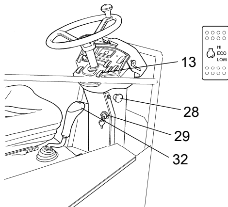
Fig. Tableau de bord 29. Interrupteur de démarrage 13. Contrôle du régime moteur 28. Arrêt d'urgence 32. Sélecteur du sens de marche
