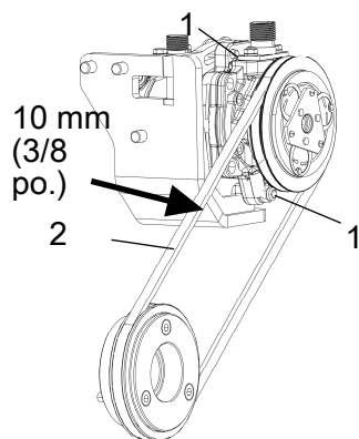
Fig. Compresseur 1. Vis 2. Tapis
