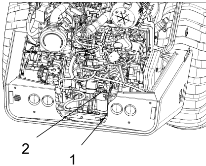
Fig. Préfiltre à carburant 1. Bouchon de vidange 2. Pompe à main
