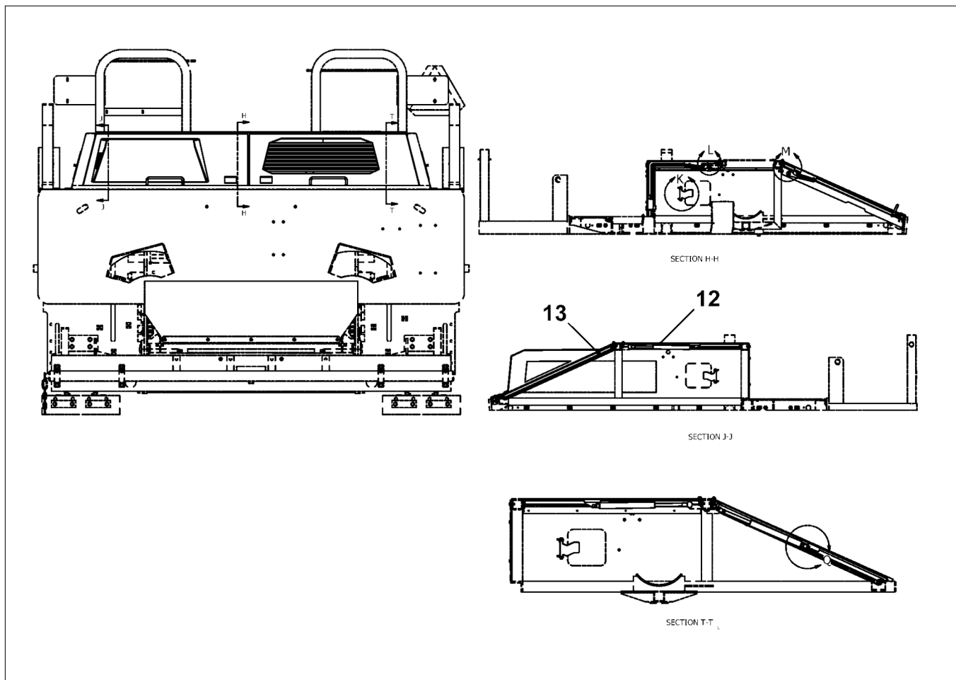
4812220020 Door
