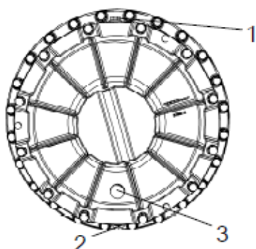
Fig. cartucho, lado esquerdo 1. Bujão de enchimento 2. Bujão de esvaziamento 3. Visor de nível
