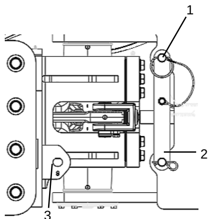
Fig. Articulação da direção na posição aberta
