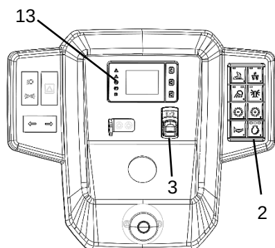
Fig. Painel de controle: 8. Seletor de velocidade; 12. Freio de estacionamento; 13. Painel luzes de advertência;
