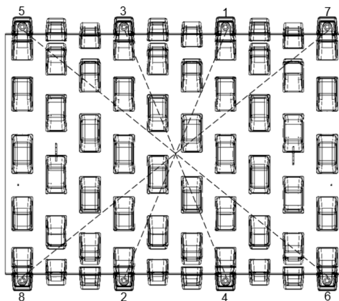
Fig. Seqüência de aperto dos parafusos casquinha
