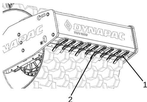
Fig. Raspador rolo com patas
