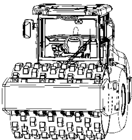
Fig. Rolo com kit casquinha montado
