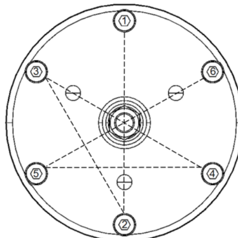
Fig. Sequência de aperto dos parafusos do eixo
