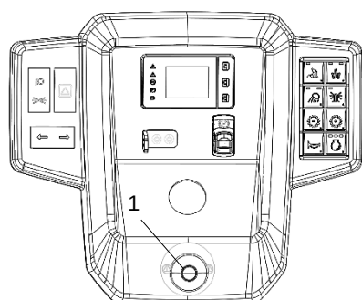
Fig. Painel de controle 1. Parada de emergência
