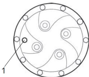
Fig. Verificação de nível – engrenagem planetária, anti-derrapagem
