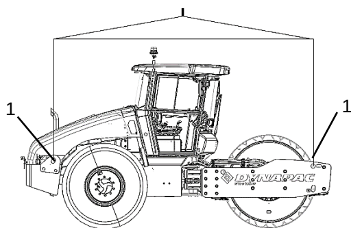
Fig. Rolo preparado para içamento 1. Placa de içamento
