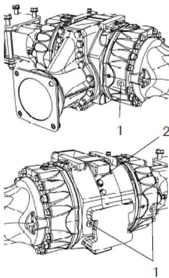
Fig. Controle do nível caixa do diferencial
