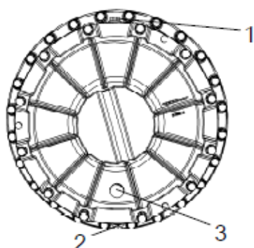
Fig. cartucho, lado esquerdo
