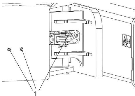
Fig. Lubrificação dos cilindros da direção
