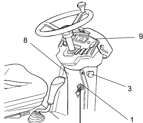
Fig. Puesto del operador
