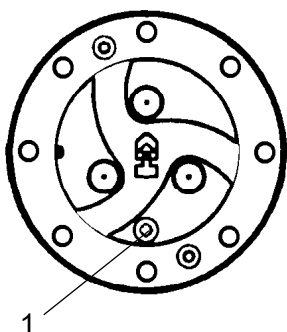
Fig. Planetario / posición de drenaje 1. Tapón
