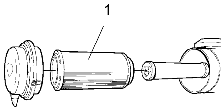
Abb. Luftfiltereinheit 1. Hauptfilter
