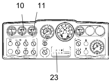
Abb. Armaturenbrett 10. Hydrauliköltemperatur (Zubehör) 11. Motoröltemperatur (Zubehör) 23. Warnleuchte, Luftfilter
