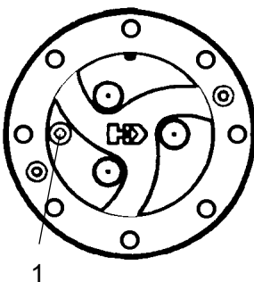
Abb. Ölstandskontrolle - Planetengetriebe 1. Ölstand/Öleinfüllschraube
