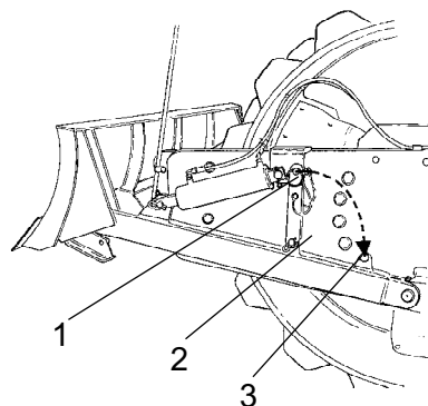
Abb. Abstreiferschild 1. Sicherungssplint 2. Sicherheitsgelenk 3. Parksperre
