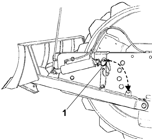
Abb. Abstreiferschild 1. Sicherungssplint
