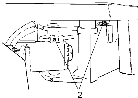
Abb. Lenkzylinder 2. Schmiernippel für Zylinderbefestigung (2 St.)
