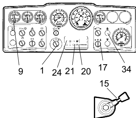
Abb. Armaturenbrett 1. Anlasserschalter 9. Voltmeter (Zubehör) 15. Drehzahlregler 17. Amplitudenwählschalter 20. Bremsleuchte 21. Öldruckleuchte 24. Ladeleuchte 34. Vorglühleuchte
