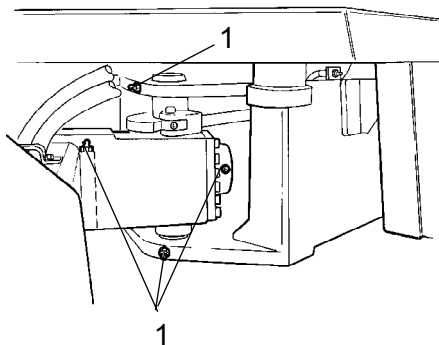
Abb. Lenkgelenk, linke Seite 1. Schmiernippel für Lenkgelenk (4 St.)
