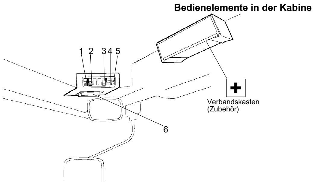
Abb. Kabinendecke, vorn
