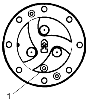
Abb. Planetengetriebe / Stellung zum Ölablassen 1. Schraube
