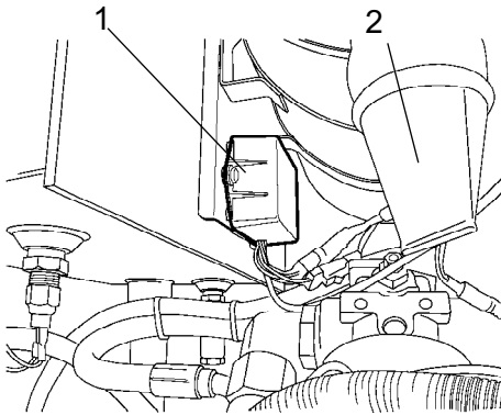
Abb. Motorraum 1. Steuerung für Motor-Vorglüheinrichtung 2. Luftfilter
