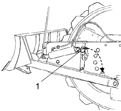
Abb. Abstreiferschild 1. Sicherungssplint
