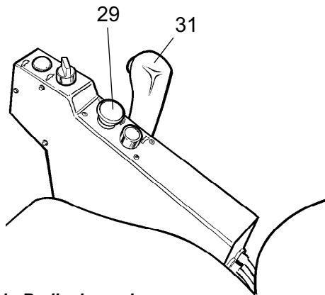
Abb. Bedienkonsole 29. Notbrems-/Feststellbremsknopf 31. Vor-/Rückwärtsfahrhebel
