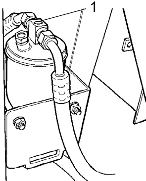
Abb. Trockenfilter 1. Schauglas
