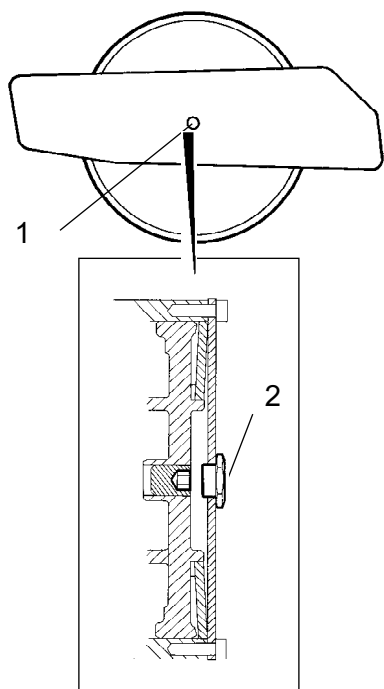
Rys. Lewa strona ramy 1. Otwór środkowy 2. Kołek środkowy
