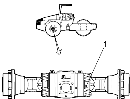
Fig. Contrôle du niveau - carter de différentiel 1. Bouchon de niveau/remplissage
