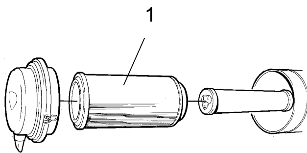
Fig. Épurateur d'air 1. Filtre principal
