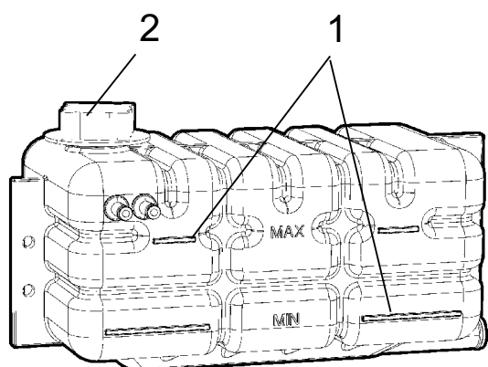
Fig. Réservoir du liquide de refroidissement
