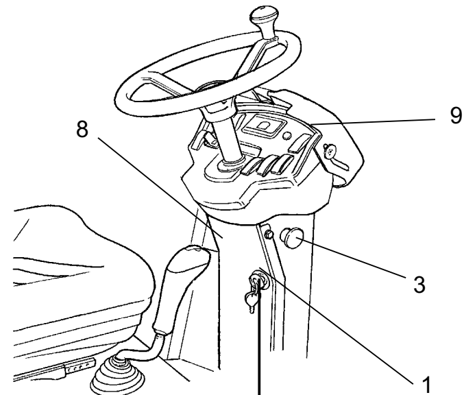
Fig. Siège du conducteur
