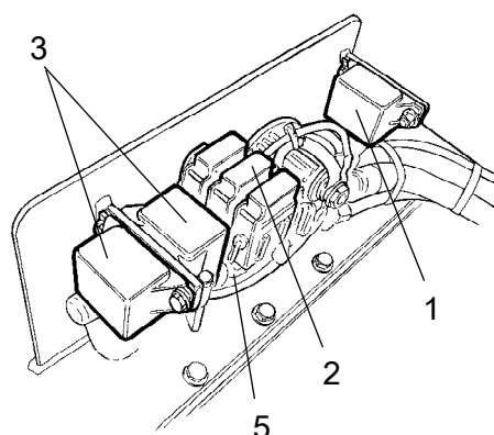
Рис. Отделение двигателя
