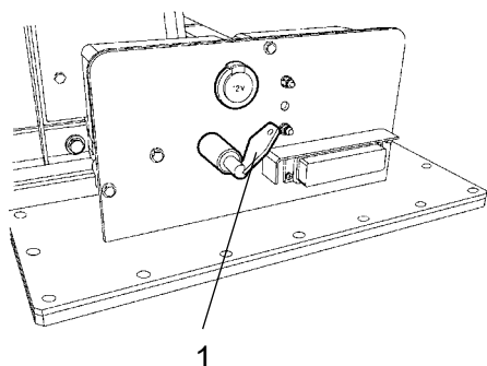
Рис. Моторное отделение 1. Главный выключатель
