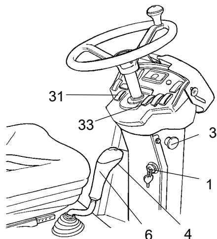
Рис. Панель управления 1. Кнопка 3. Аварийный выключатель 4. Переключатель вкл./выкл. 6. Рычаг прямого/обратного хода 31. Выключатель стояночного тормоза 33. Регулятор частоты оборотов
