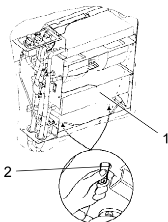
Рис. Автоматический кондиционер 1. Элемент системы охлаждения 2. Сливной клапан (x2)
