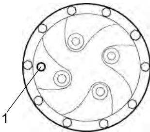
Рис. Проверка уровня - планетарная передача, без вращения
