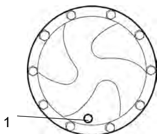
Рис. Слив масла - планетарная передача
