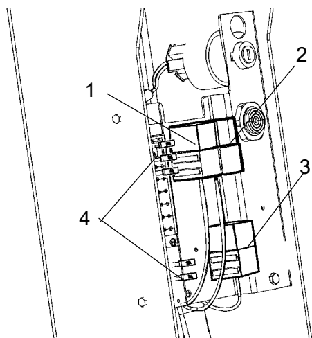
Рис. Плата системы управления 1. Реле прерывателя сигналов 2. Реле стоп-сигналов 3. Реле рабочего освещения 4. Блоки предохранителей
