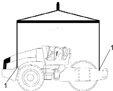
Рис. Подготовленный к подъему каток
