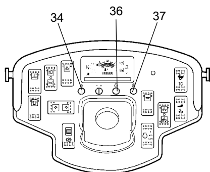
Рис. Приборная панель 34. Диагностика двигателя вкл/выкл 36. Индикатор серьезной неисправности 37. Индикатор некритической ошибки
