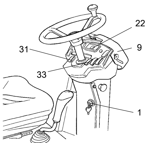
Рис. Приборная панель 1. Выключатель стартера 9. Защитная рамка для приборов 22. Панель сигнальных ламп 31. Выключатель стояночного тормоза 33. Регулятор частоты оборотов
