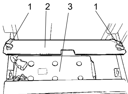
Рис. Кронштейн аккумулятора
