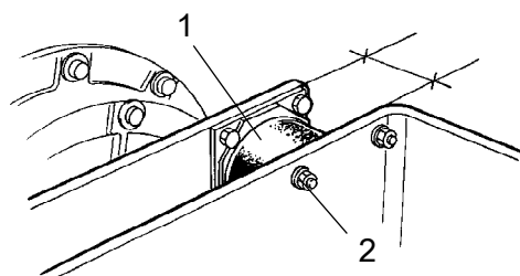
Рис. Валец, сторона вибрации 1. Резиновый элемент 2. Крепежные винты
