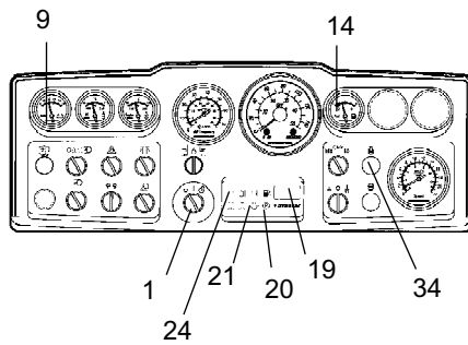
Fig. Instrumentenpaneel 1. Startschakelaar 9. Voltmeter (accessoire) 14. Brandstofmeter 19. Urenmeter 20. Remlampje 21. Oliepomp lampje 24. Opladlampje 34. Voorverwarmingslampje
