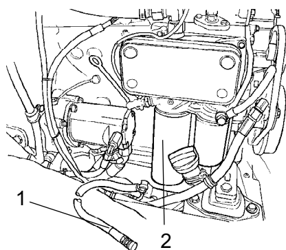
Fig. Linkerzijde van de motor 1. Aftapplug 2. Oliefilter
