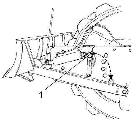
Рис. Выравнивающее лезвие 1. Шплинт
