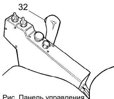
Рис. Панель управления 32. Выключатель вибрации вкл./выкл.
