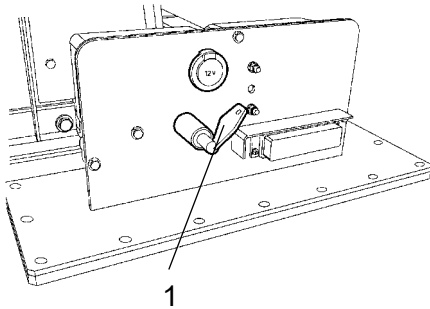
Fig. Compartimento del motor 1. Interruptor de aislamiento de la batería
