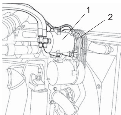
Obr. Motorový priestor 1. Kompresor 2. Hnací pás
