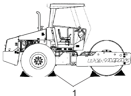
Obr. Umiestnenie 1. Klíny
