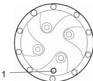
Obr. Vypúšťanie oleja - planétová prevodovka, voliteľná 1. Zátka na kontrolu hladiny/Pniaca zátka
