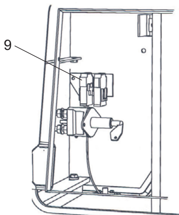
Obr. Odpojovač batérie/poistková skrinka v priestore chladiča. 9. Poistka
