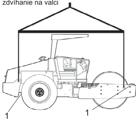
Obr. Valec pripravený na zdvíhanie 1. Štítok s údajmi pre zdvíhanie
