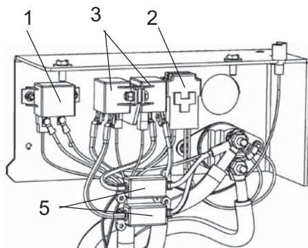
Obr. Kryt motora
