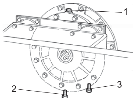
Obr. Pravá strana bubna 1. Plniaca zátku 2. Výpustná zátku 3. Zátku na kontrolu hladiny
