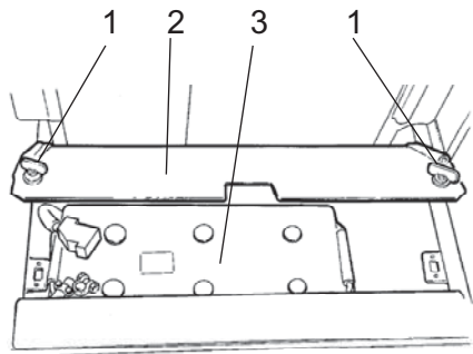
Obr. Umiestnenie batérie 1. Rýchlopínacie skrutky 2. Kryt batérie 3. Batéria
