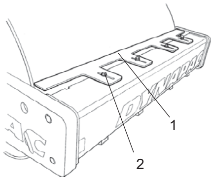
Obr. Škrabáky 1. Čepele škrabáka 2. Skrutky (4)
