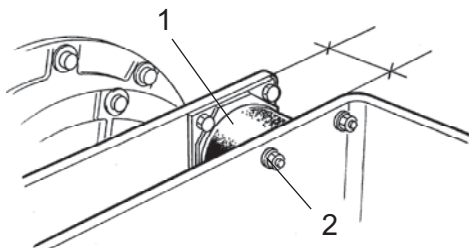
Obr. Bubon, strana s vibračným systémom 1. Gumený prvok 2. Upevňovacie skrutky
