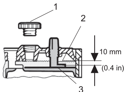
Obr. Hladina elektrolytu v batérii
