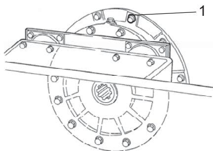
Obr. Bubon 1. Ventilačná skrutka
