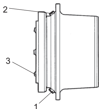
Obr. Prevodovková skriňa bubna 1. Vypúšťacia zátka 2. Plniaca zátka 3. Zátka na kontrolu hladiny
