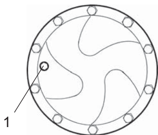
Obr. Kontrola úrovne - planétová prevodovka, štandardná 1. Zátka na kontrolu hladiny/Plniaca zátka
