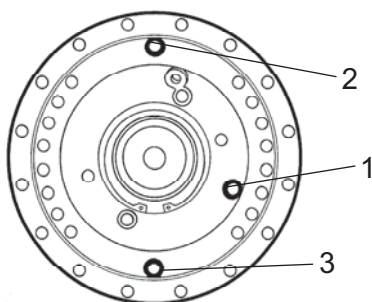
Obr. Kontrola úrovne oleja - prevodková skriňa bubna 1. Zátka na kontrolu hladiny 2. Plniaca zátka 3. Výpustná zátka
