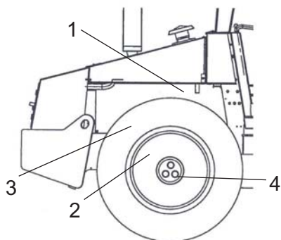
Obr. Pravá strana stroja 1. čerpadlo riadenia 2. Zadná náprava 3. Zavesenie motora 4. Matice kolesa
