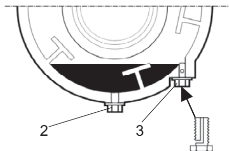
Obr. Vložka bubna 2. Vypúšťacia zátku 3. Zátku na kontrolu hladiny
