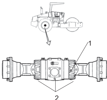
Obr. Zadná náprava 1. Zátka na kontrolu hladiny/Plniaca zátka 2. Výpustné zátka
