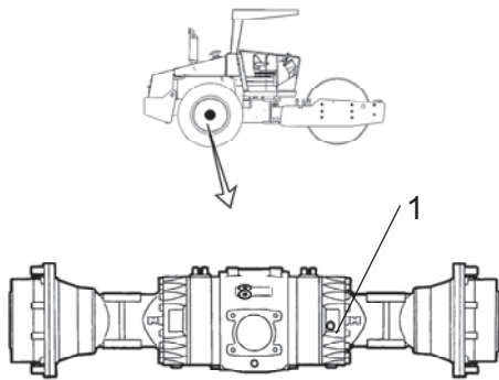
Obr. Kontrola úrovne - kryt diferenciálu 1. Zátka na kontrolu hladiny/Plniaca zátka
