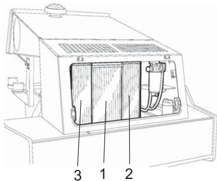
Obr. Priestor motora 1. Chladič vody 2. Chladič plniaceho vzduchu 3. Chladič hydraulickej kvapaliny
