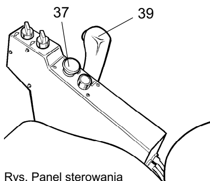
Rys. Panel sterowania 37. Pokrętko hamulca rezerwowego/postojowego 39. Dźwignia jazdy do przodu / do tyłu
