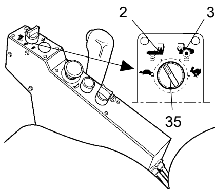
Fig. Panel de control 35. Selector de velocidad, cilindro/ruedas (opcional) 2. Posición 2 3. Posición 3
