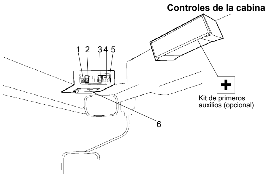
Fig. Techo de la cabina, parte frontal
