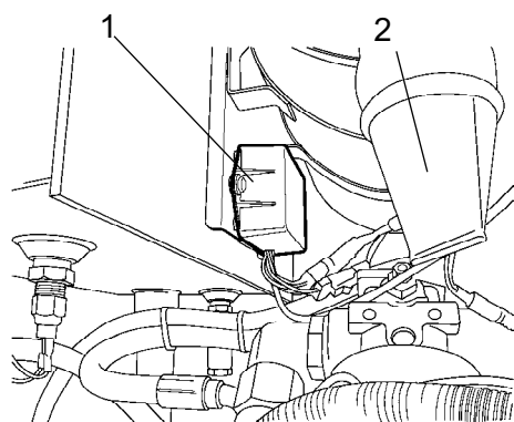
Рис. Отсек двигателя
