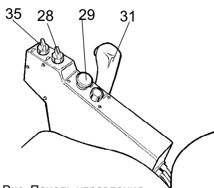
Рис. Панель управления 28. Переключатель скоростей, задняя ось 29. Кнопка заднего хода/стояночного тормоза 31. Рычаг прямого/обратного хода 35. Переключатель скоростей, валец
