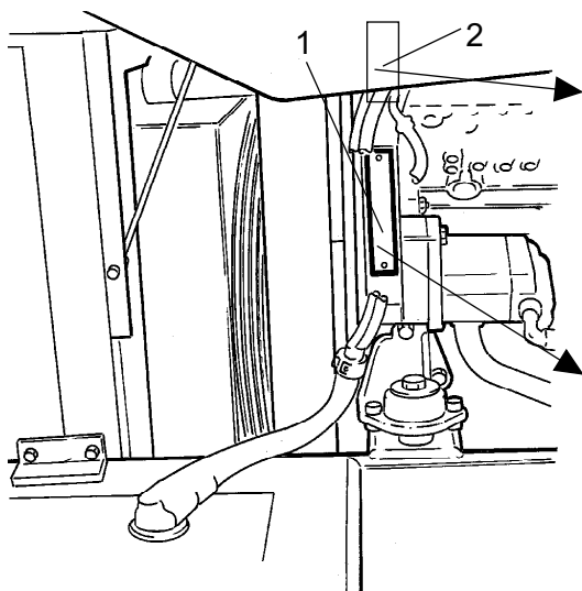
Рис. Двигатель 1. Табличка с типом 2. Табличка ЕРА (США)
