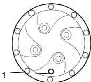
Fig. Réducteur planétaire/position de vidange
