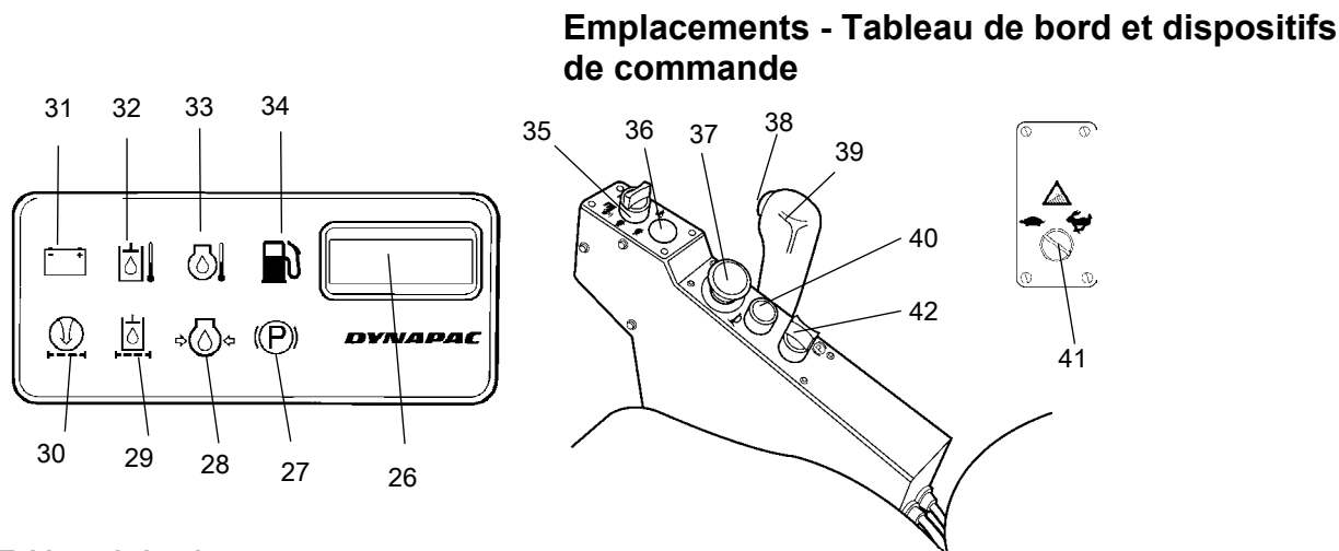
Fig. Tableau de bord
