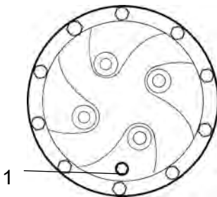
Εικ. Πλανητικό σύστημα γραναζιών/θέση αποστράγγισης
