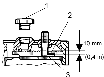
Εικ. Στάθμη ηλεκτρολύτη στην μπαταρία
