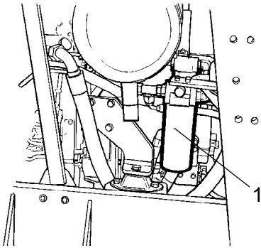
Рис. Отсек двигателя 2. Фильтр гидравлической жидкости (x2)
