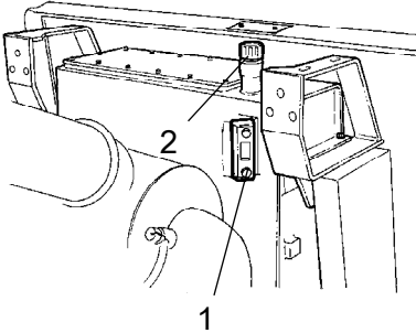
Şekil Hidrolik sıvısı deposu 1. Gözetleme camı 2. Doldurma borusu
