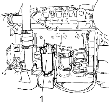
Şekil Motor bölmesi 1. Yakıt ön filtresi
