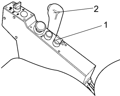
Şekil Kumanda paneli 1. Park freni düğmesi 2. İleri/geri hareket kolu
