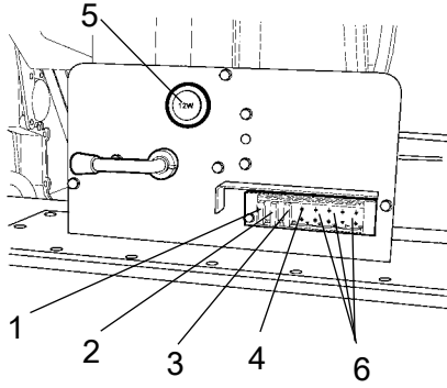
Şekil Motor bölümü
