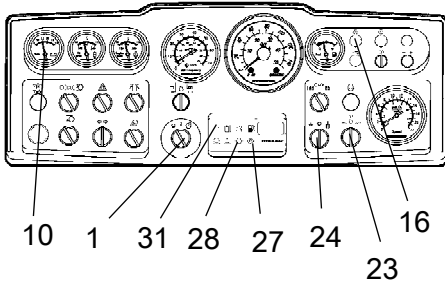
Şekil Gösterge paneli 1. Marş anahtarı 10. Voltmetre (İsteğe bağlı). 16. Ön ısıtma lambası 23. Motor hızı kumandası 24. Salınım yüksekliği seçici 27. Fren lambası 28. Yağ basıncı lambası 31. Şarj lambası
