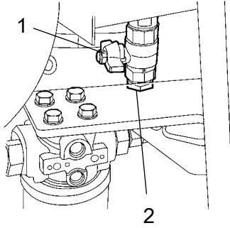
Şekil Hidrolik sıvısı deposunun altı 1. Boşaltma tapası 2. Tapa
