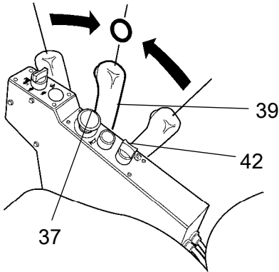
Şekil Kumanda paneli 37. Acil durdurma 39. İleri/Geri kolu 42. Park freni düğmesi
