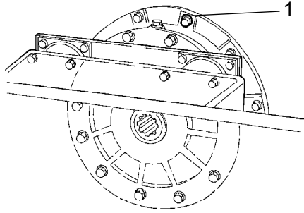
Şekil Silindir 1. Havalandırma vidası
