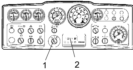
Şekil Gösterge paneli 1. Marş anahtarı 2. Uyarı lambaları paneli
