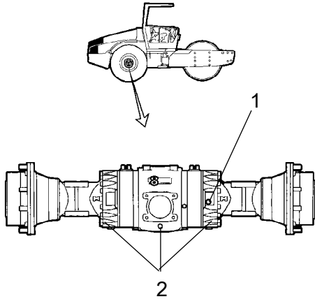
Şekil Arka dingil 1. Seviye/Doldurma tapası 2. Boşaltma tapaları
