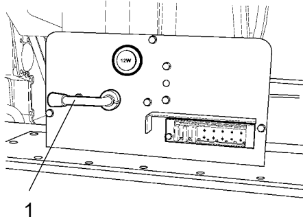
Şekil Motor bölümü 1. Ana şalter
