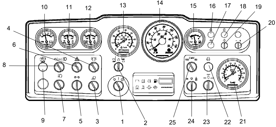
Şekil Gösterge aletleri ve kumanda paneli
