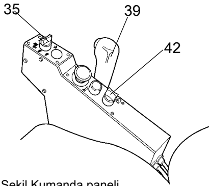
Şekil Kumanda paneli 35. Hız seçici 39. İleri/Geri kolu 42. Park freni düğmesi
