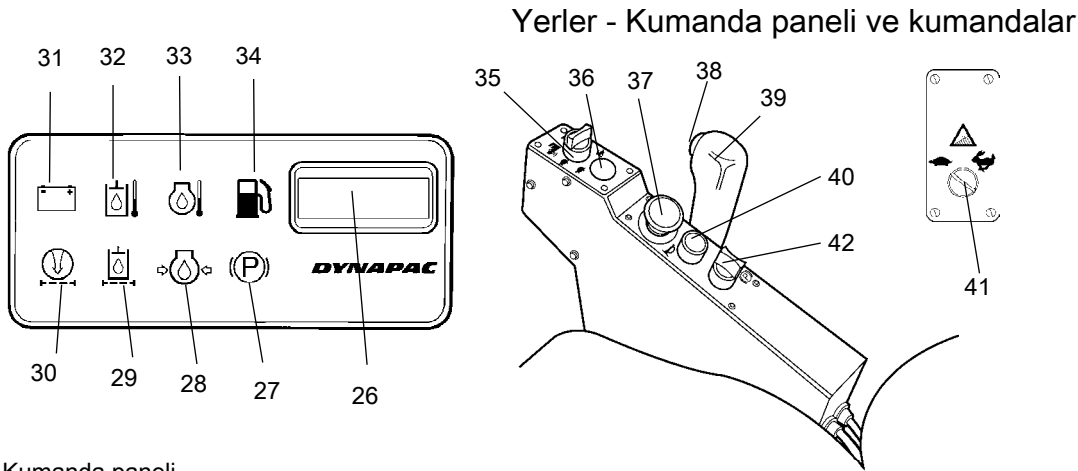
Şekil Kumanda paneli
