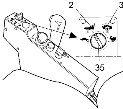
Şekil Kumanda paneli 35. Hız seçici 2. Konum 2 3. Konum 3
