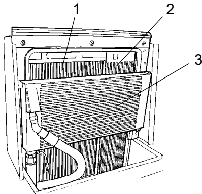
Şekil Motor bölümü 1. Su soğutucu 2. Besleme havası soğutucu 3. Hidrolik sıvısı soğutucu
