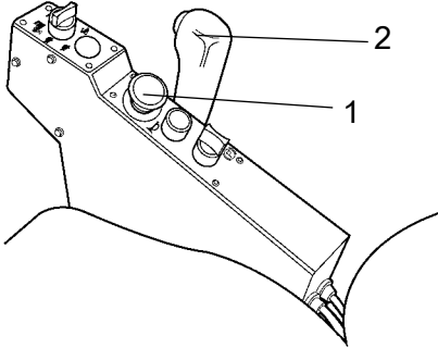
Şekil Kumanda paneli 1. Park freni düğmesi 2. İleri/geri hareket kolu
