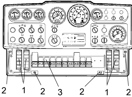
Şekil Gösterge paneli 1. Sigorta kutuları (4) 2. Hızlı vidalar 3. Röleler
