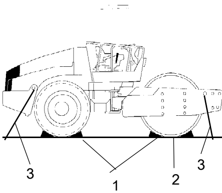
Şekil Nakliye 1. Takoz 2. Blok koyun 3. Bağlama teli
