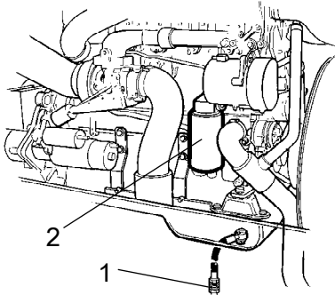
Şekil Motorun sol tarafı 1. Boşaltma tapası 2. Yağ filtresi
