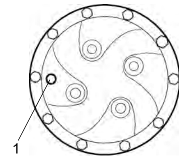
Şekil. Seviye kontrolü - planeter dişli 1. Seviye/Doldurma tapası
