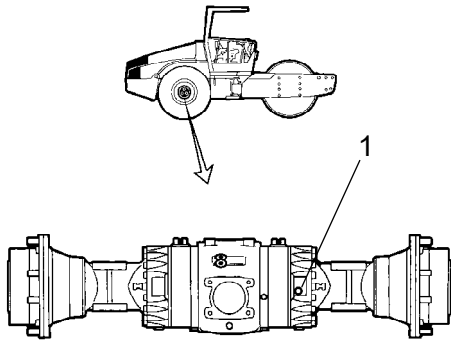
Şekil. Seviye kontrolü - diferansiyel muhafazası 1. Seviye/Doldurma tapası
