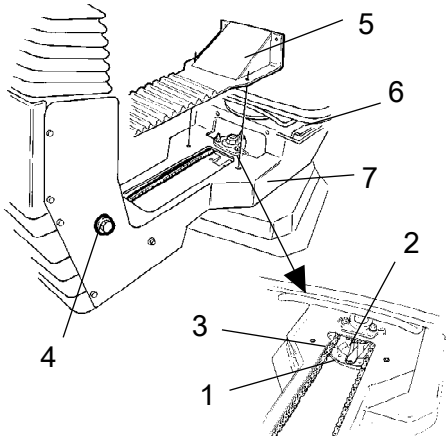
Şekil Koltuk yatağı
