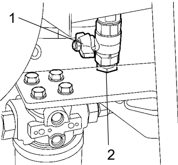
Şekil Hidrolik sıvısı deposunun altı 1. Boşaltma tapası 2. Tapa
