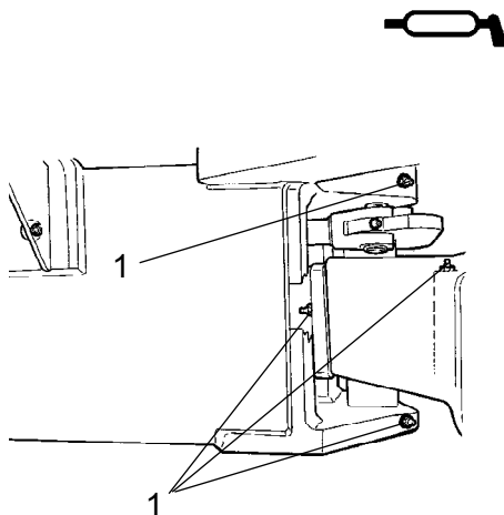
Fig. Articulation, côté droit 1. Graisseurs, articulation (4)
