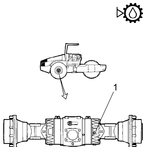
Fig. Contrôle du niveau - carter de différentiel 1. Bouchon de niveau/remplissage
